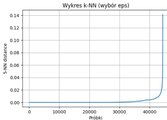
Rysunek 13: Wykres 5-NN dla danych z wektorem \vec{f}_2 – wybór parametru \text{eps} .
