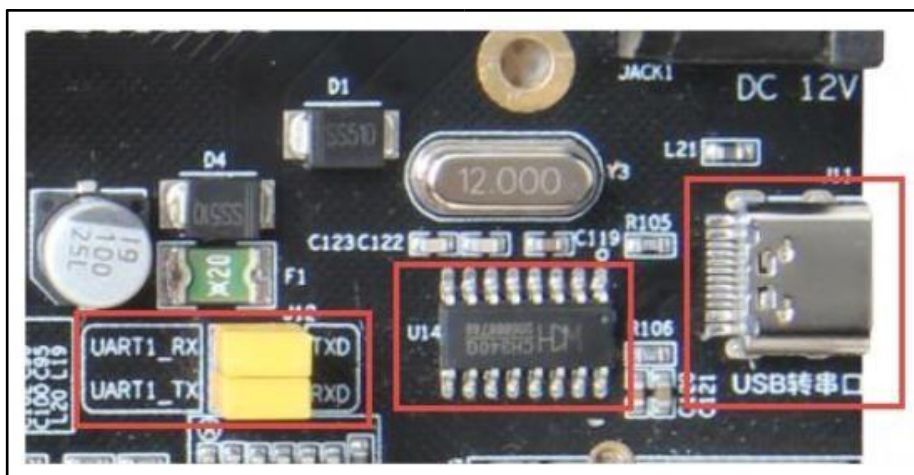
图 3.4-26 USB 转串口实物图
