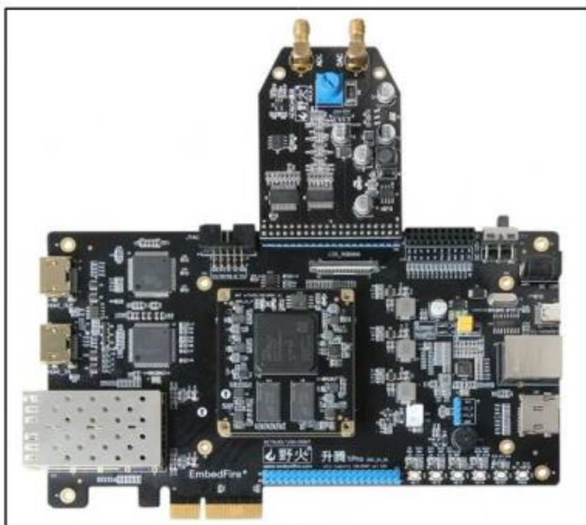
图 3.4-39 野火高速 AD/DA 模块与开发板连接
