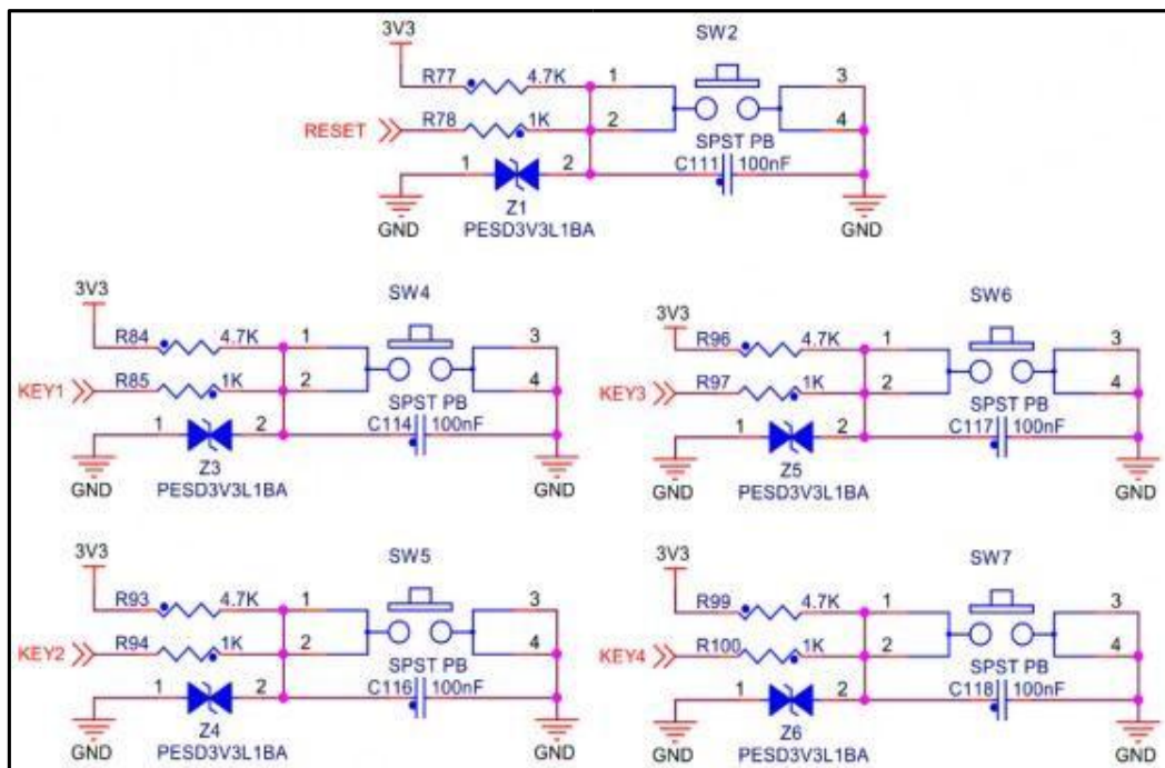
图 3.4-30 按键原理图
