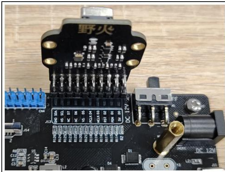
图 3.4-18 摄像头与开发板连接
