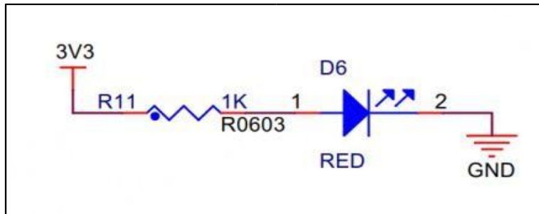
图 3.4-31 电源指示灯原理图
