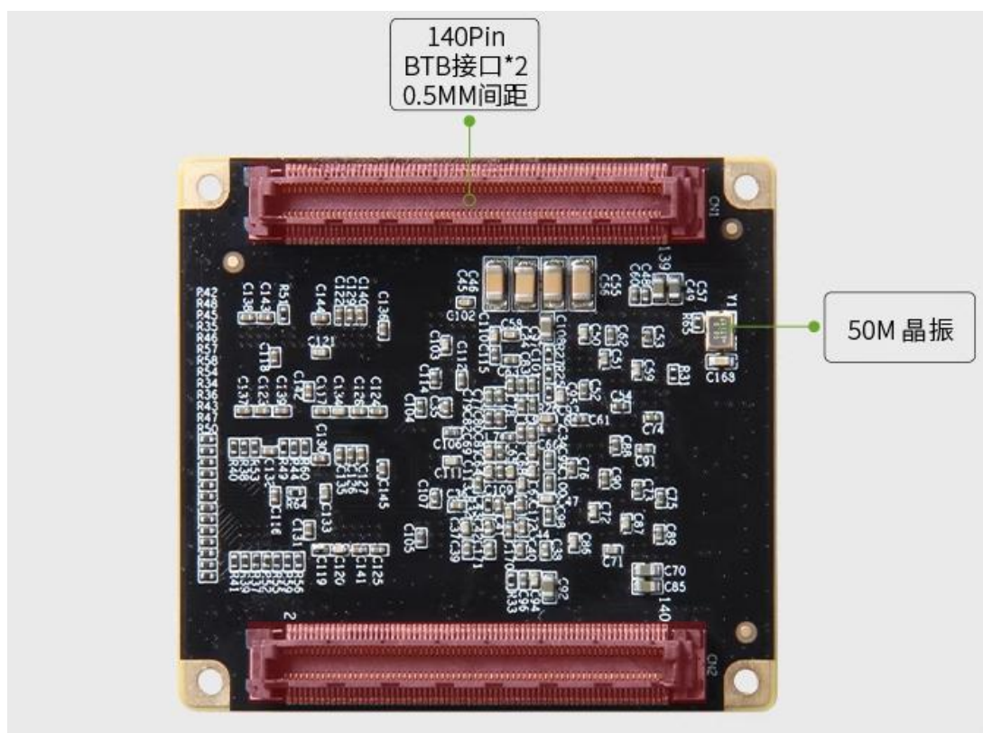
图 2.1-2 升腾_Pro 核心板背面视图
