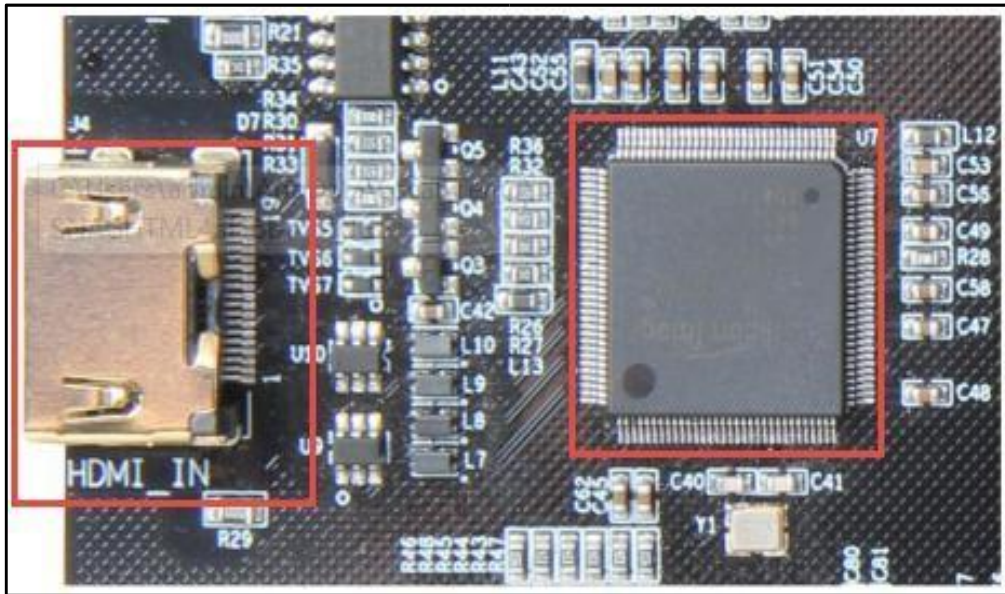
升腾 Pro 底板上的 HDMI 输入接口以及解码芯片如图 3.4-8 所示，接口类型为 Type A 型。
