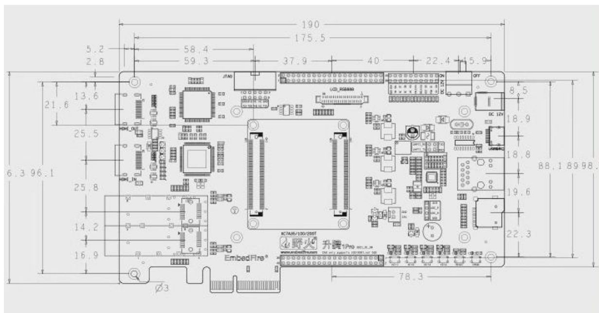
图 3.2-1 升腾_Pro 开发板底板正面机械尺寸图
