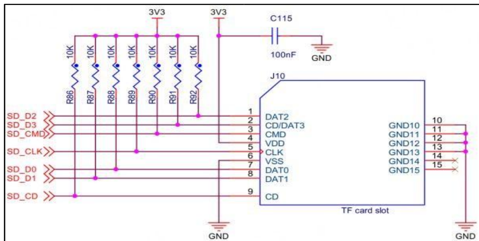
图 3.4-19 SD 卡接口原理图
