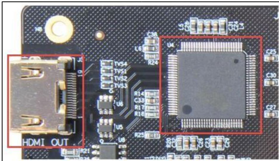
图 3.4-6 HDMI 接口实物图
