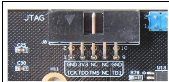
图 3.4-22 JTAG 接口实物图
