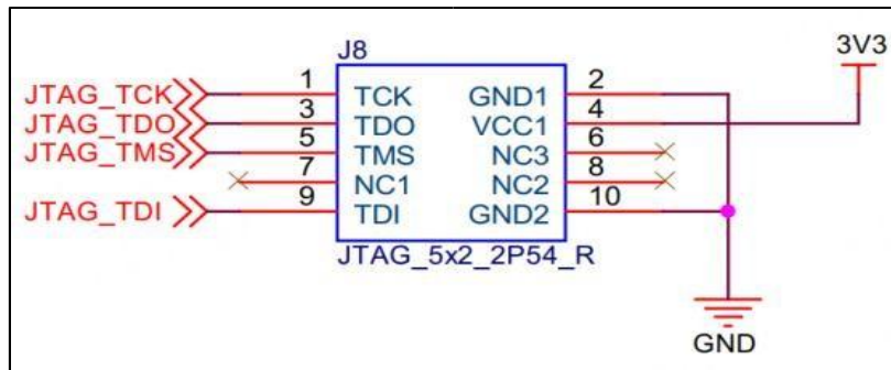
图 3.4-21 JTAG 接口原理图
