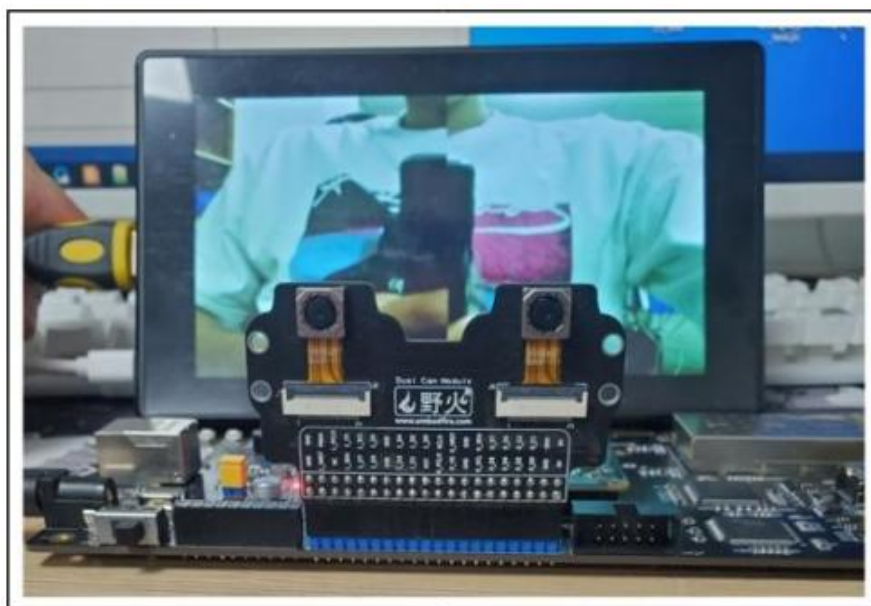
图 3.4-40 野火双目 OV5640 摄像头模块与开发板连接
