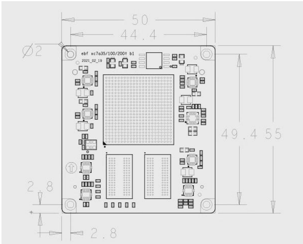
图 2.2-1 升腾_Pro 核心板正面机械尺寸图
