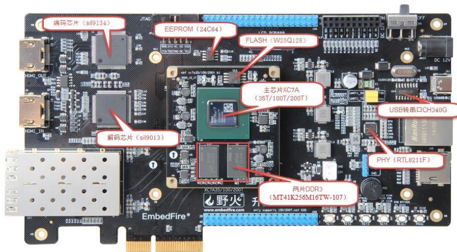
图 3.4-41 升腾 Pro 芯片位置图
