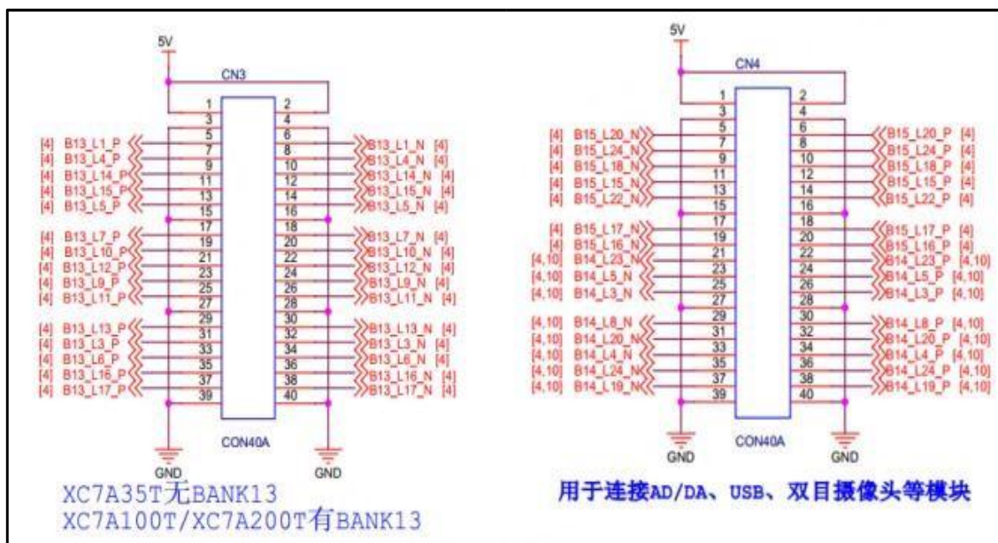
图 3.4-37 拓展 IO 口原理图
