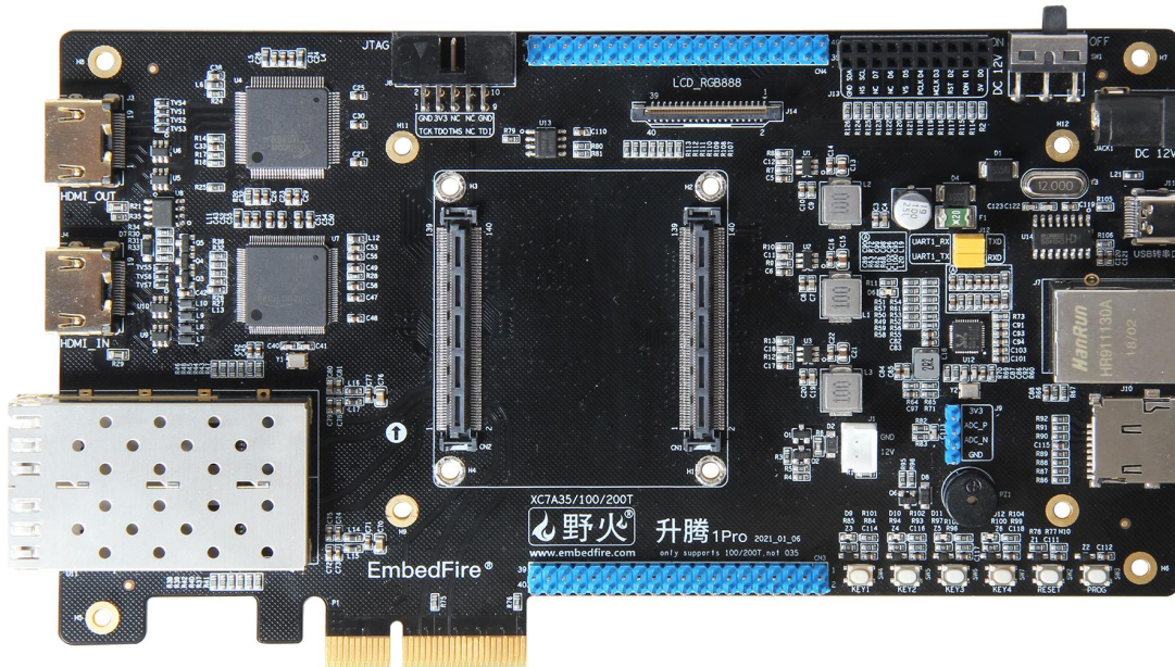
图 3.1-1 升腾_Pro 开发板底板正面视图
