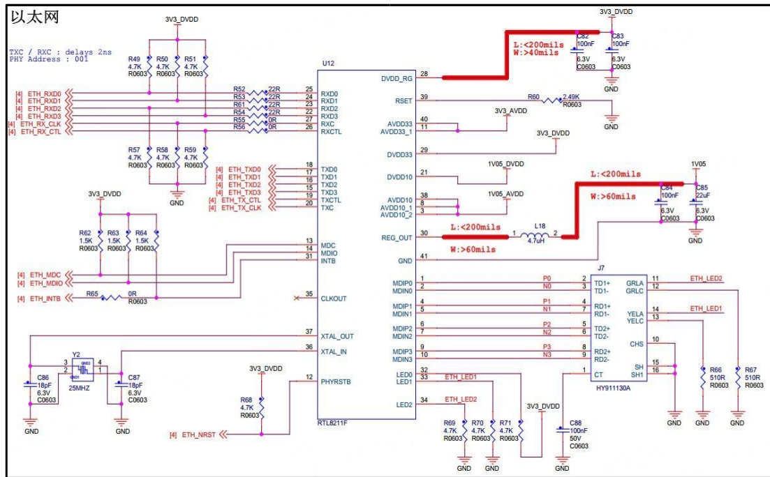
图 3.4-12 以太网部分原理图
