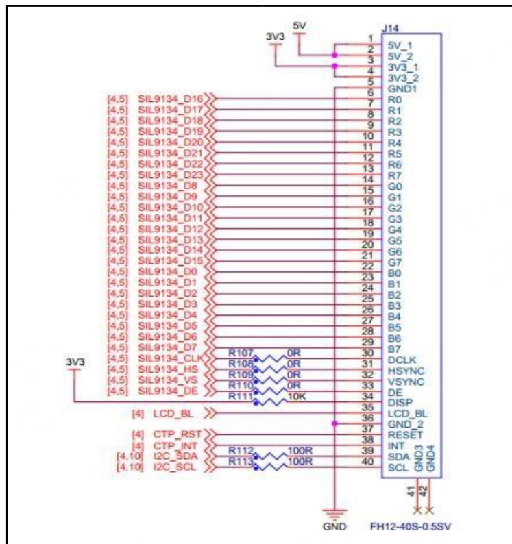
图 3.4-34 TFT_LCD 接口原理图
