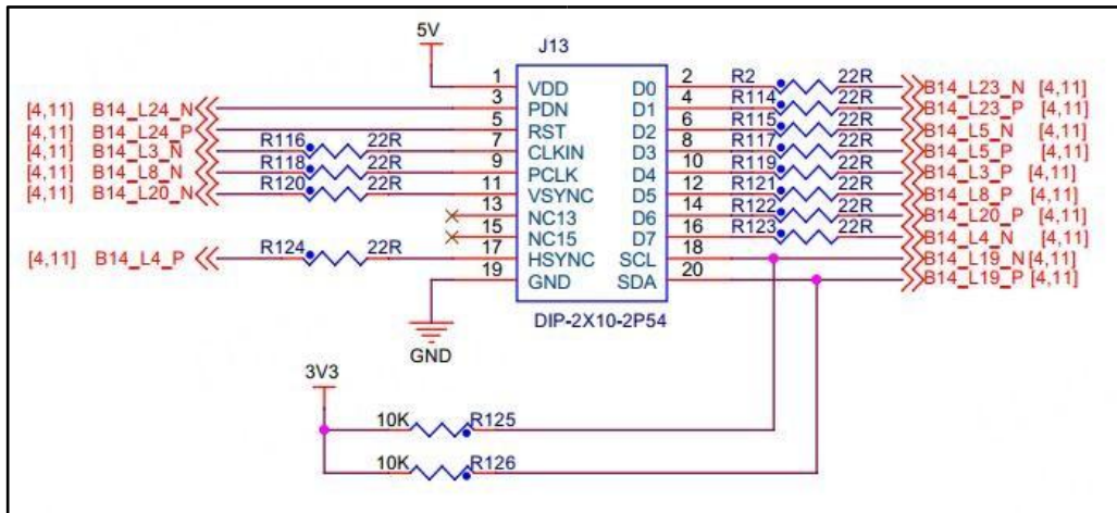
图 3.4-16 摄像头接口原理图
