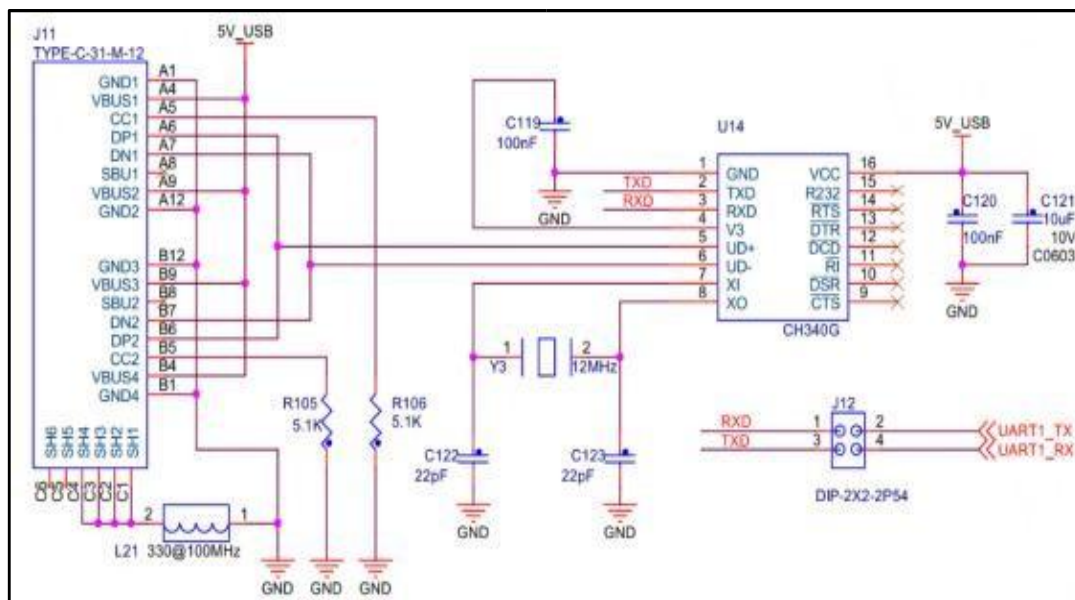
图 3.4-25 USB 转串口原理图
