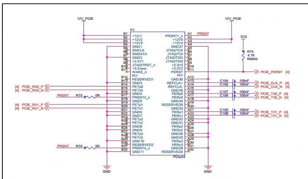
图 3.4-14 PCIe 接口原理图
