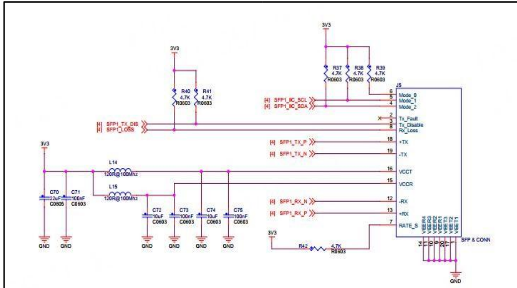
图 3.4-9 光纤接口 1 原理图
