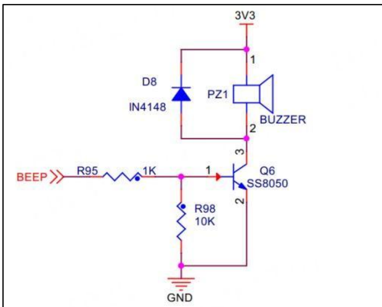
图 3.4-23 无源蜂鸣器原理图
