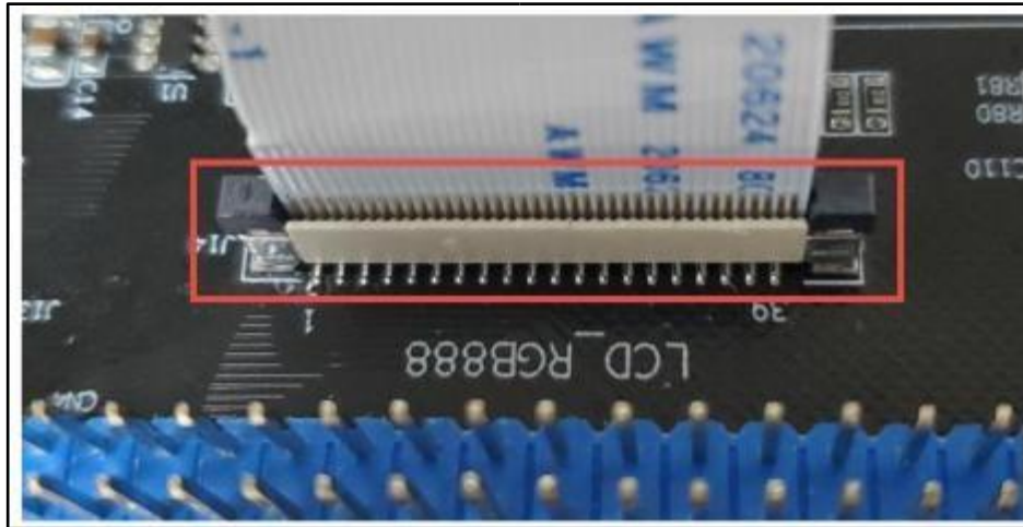
图 3.4-36 野火 TFT_LCD 接法
