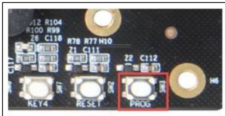
图 3.4-29 FPGA 重配置按键实物图
