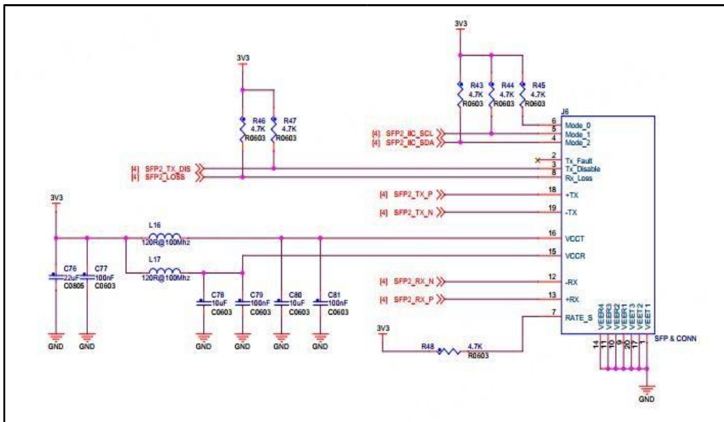
图 3.4-10 光纤接口 2 原理图
