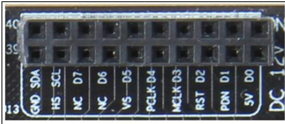
图 3.4-17 摄像头接口实物图
