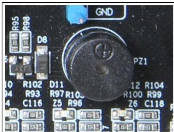
图 3.4-24 无源蜂鸣器实物图
