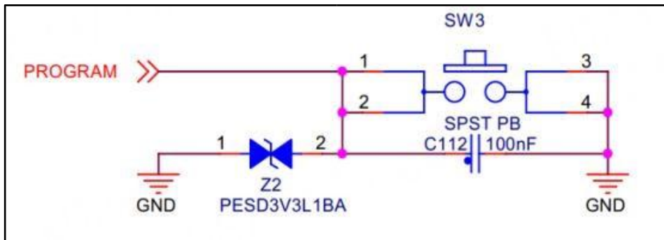
图 3.4-27 FPGA 重配置按键原理图
