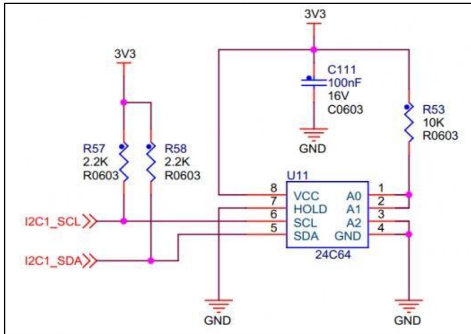
图 3.4-3 开发板 EEPROM 原理图
