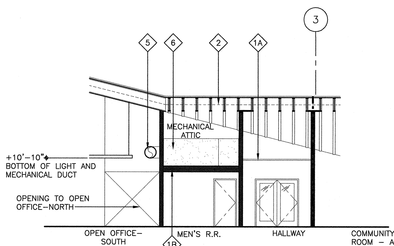
3 Section 3-3 SCALE: 1/8" = 1'-0"
