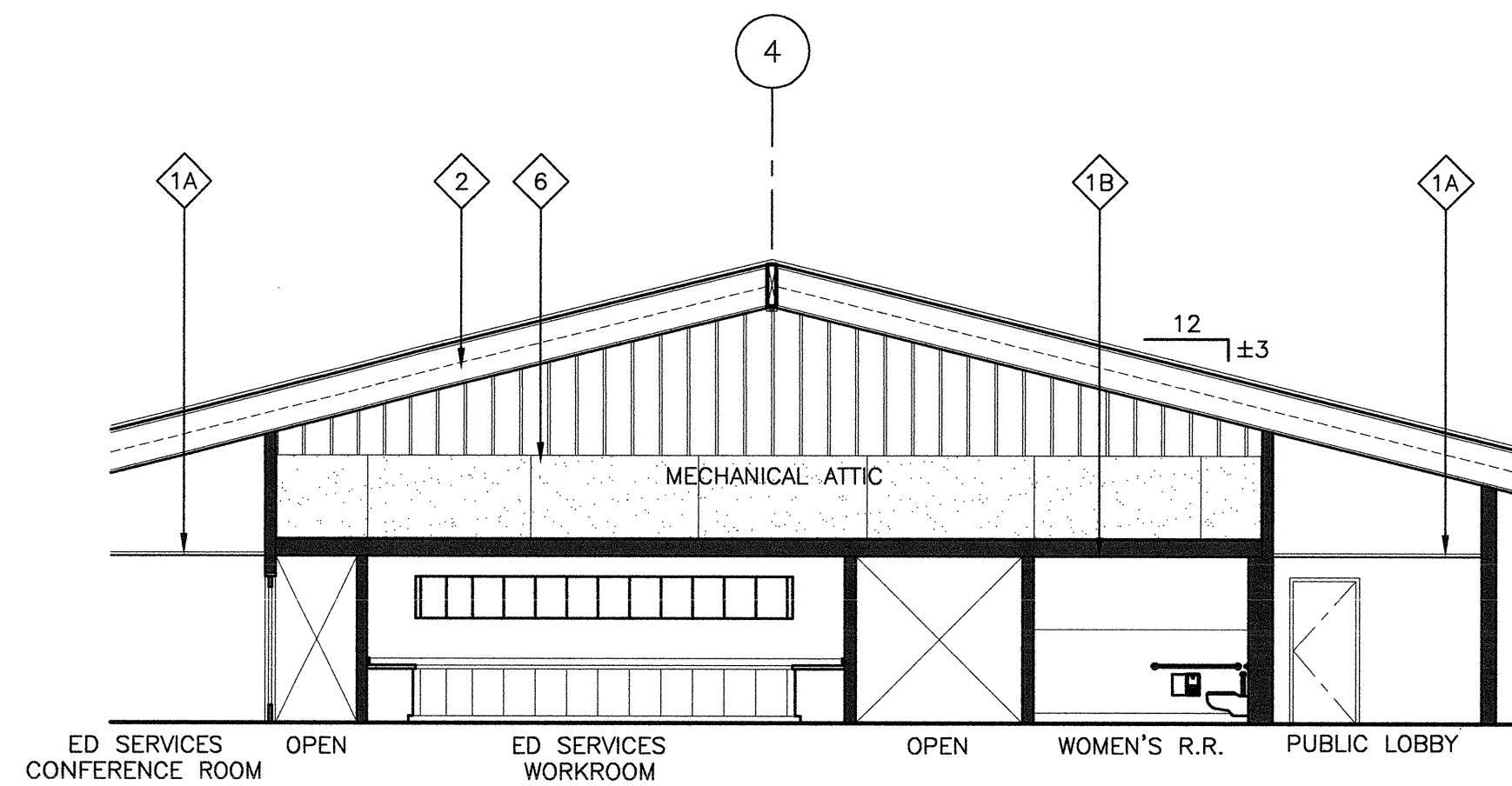
4 Section 4-4 SCALE: 1/8" = 1'-0"
