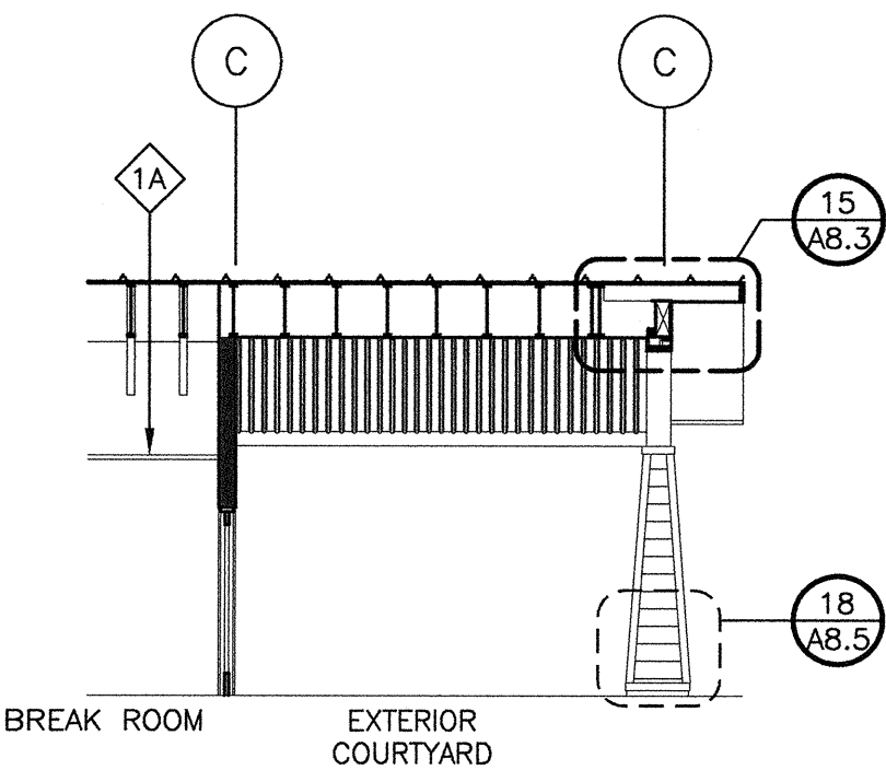
7 Section 7-7 SCALE: 1/8" = 1'-0"
