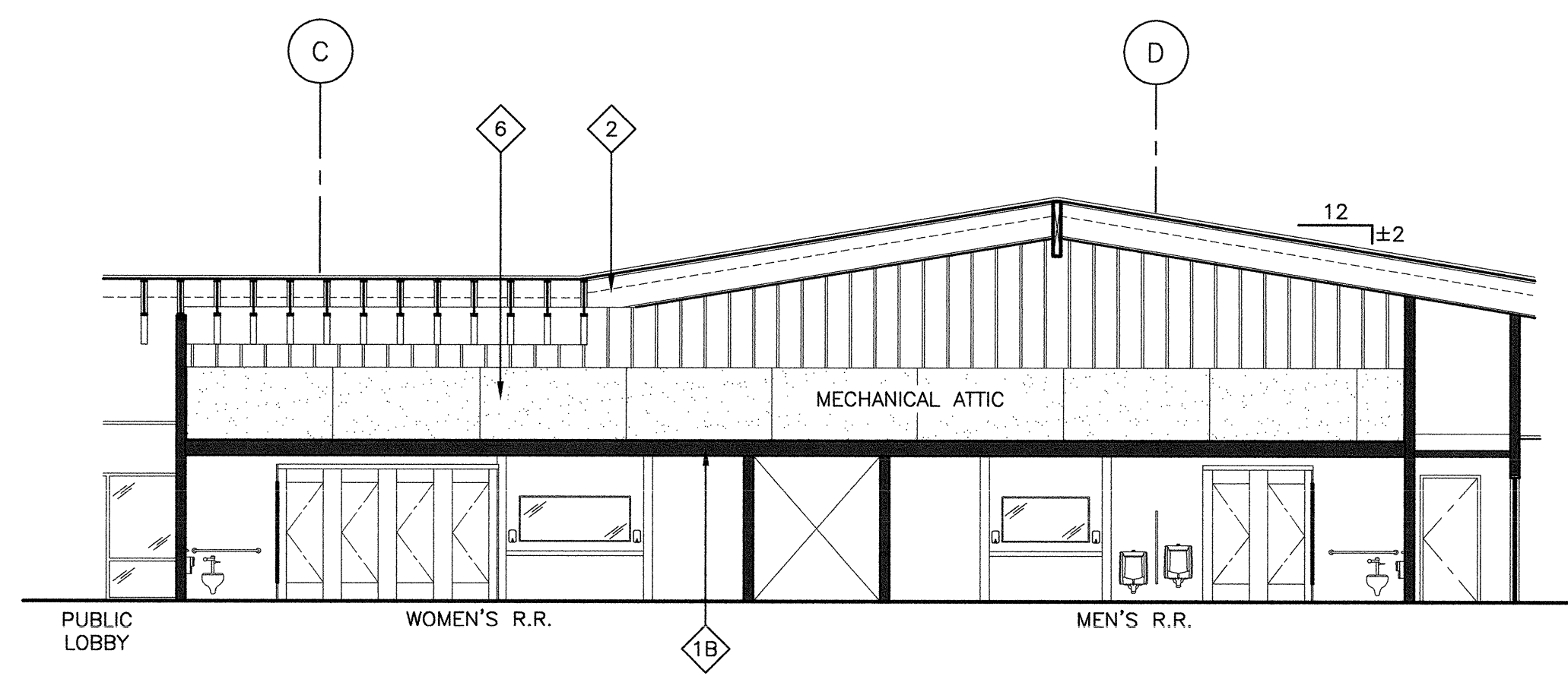
5 Section 5-5 SCALE: 1/8" = 1'-0"
