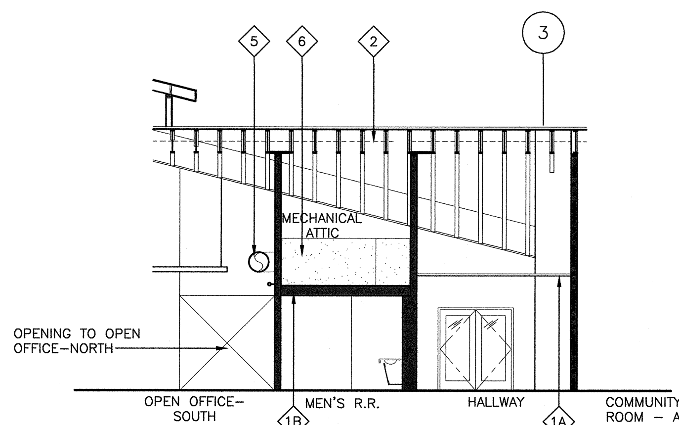
2 Section 2-2 SCALE: 1/8" = 1'-0"
