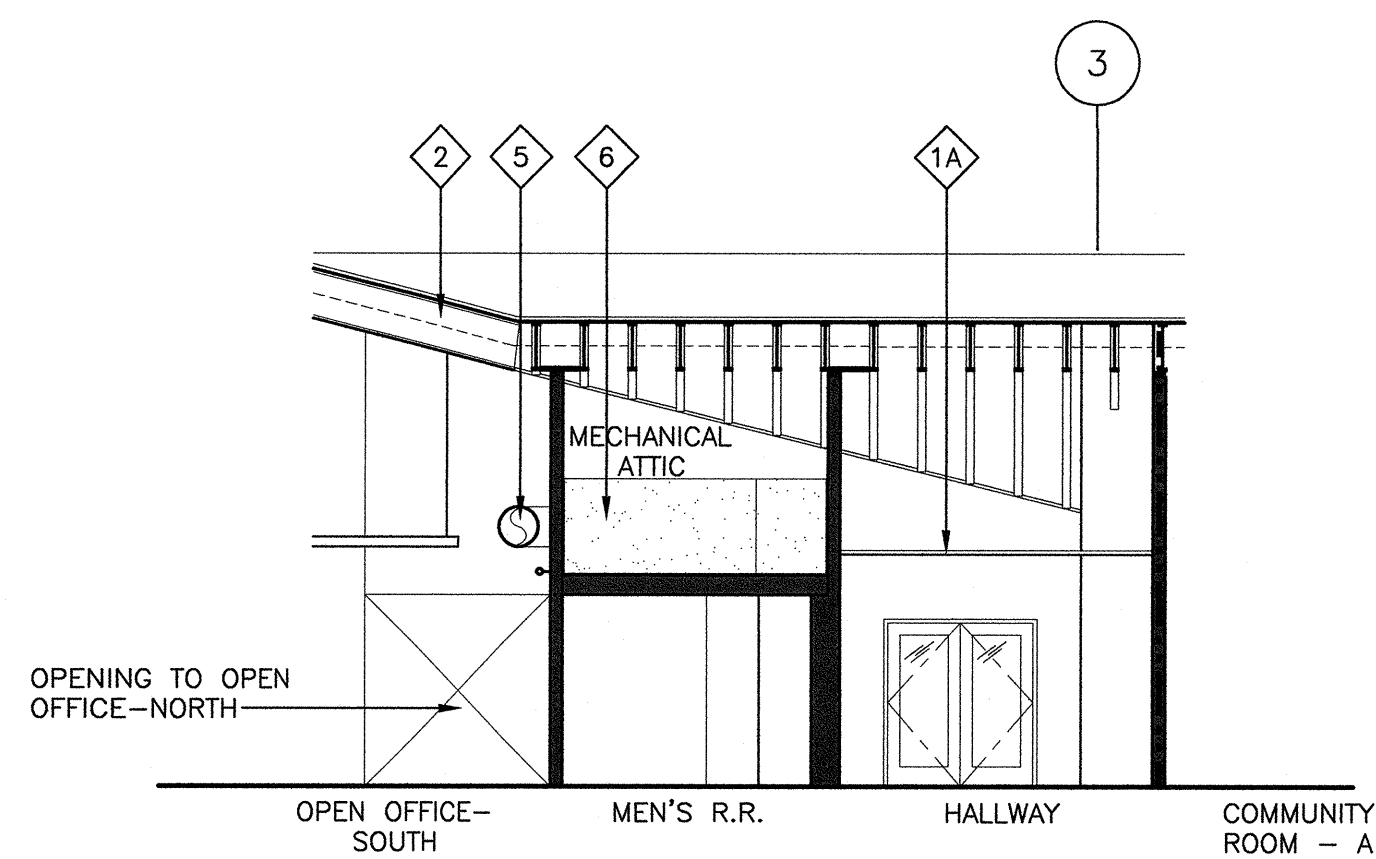
1 Section 1-1 SCALE: 1/8" = 1'-0"
