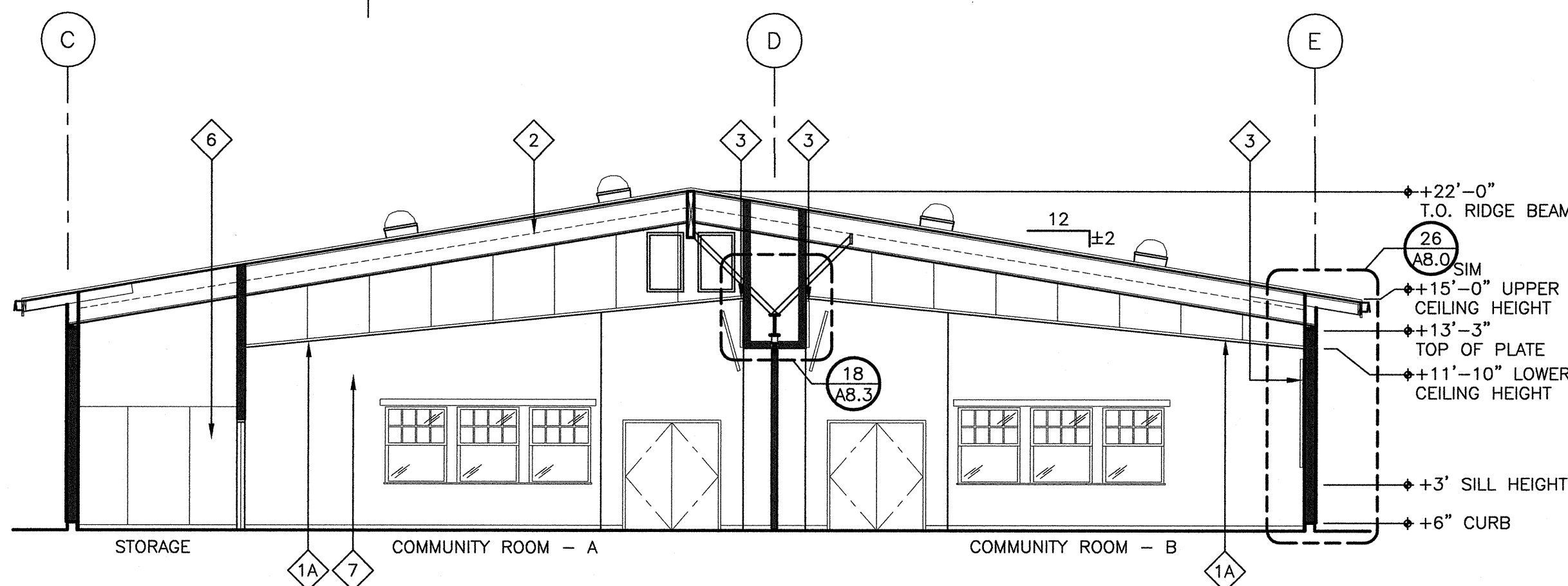
1 Section 1-1 SCALE: 1/8" = 1'-0"
