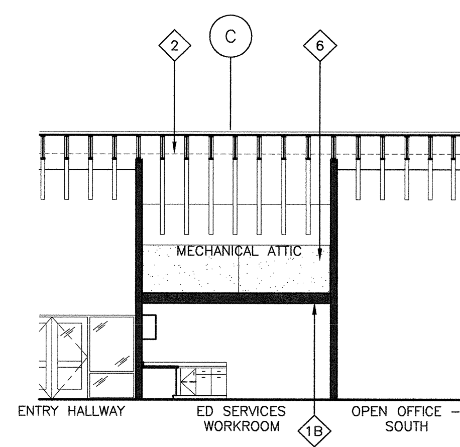
6 Section 6-6 SCALE: 1/8" = 1'-0"
