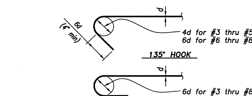
135° HOOK (14)
