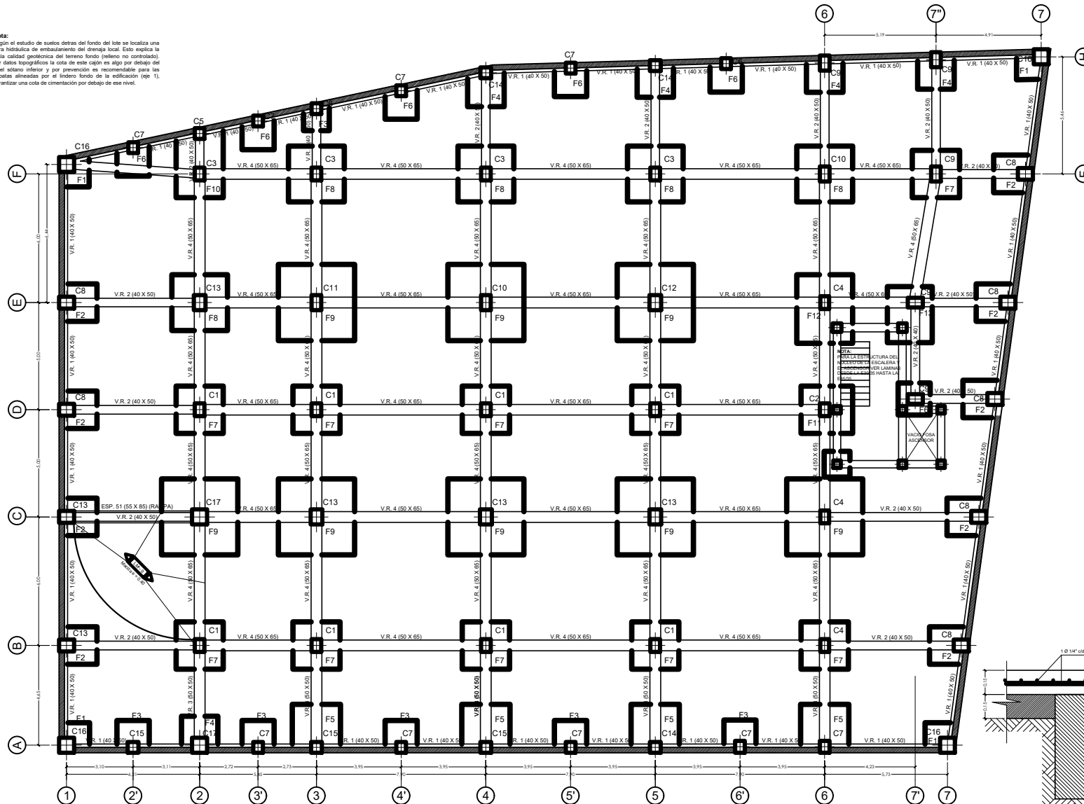
Planta índice fundaciones _____ Esc. 1: 75
