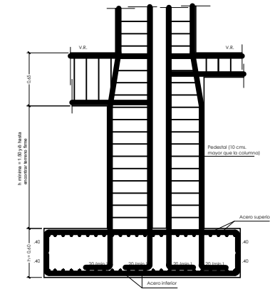
Detalle fundación F11
