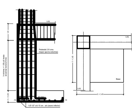
Detalle fundación F1
