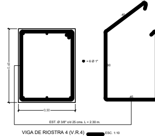
VIGA DE RIOSTRA 4 (V.R.4)
