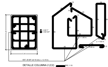
DETALLE COLUMNA 2 (C2)
