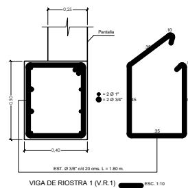
VIGA DE RIOSTRA 1 (V.R.1)
