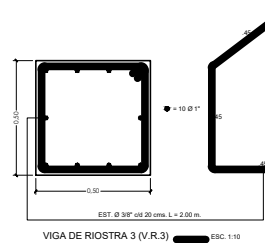
VIGA DE RIOSTRA 3 (V.R.3)
