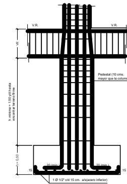
Detalle fundación F6
