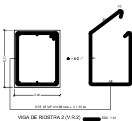
VIGA DE RIOSTRA 2 (V.R.2)
