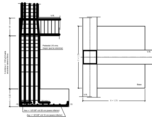
Detalle fundación F2
