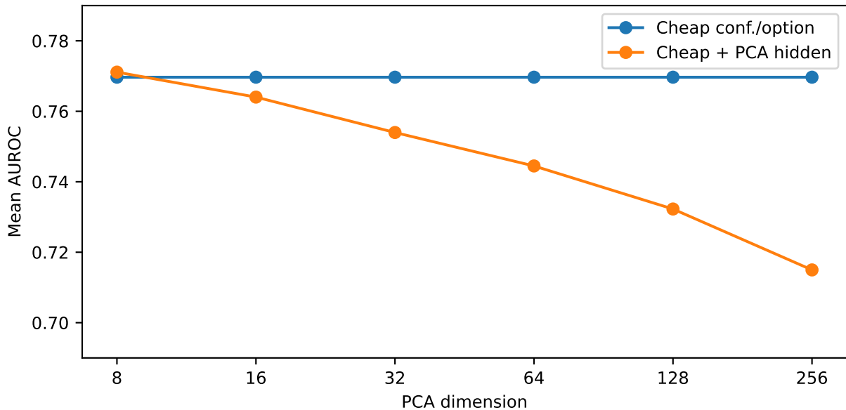
PCA dimension sensitivity
