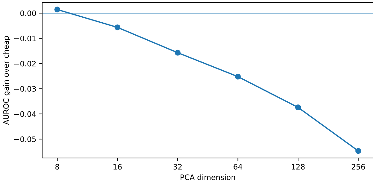
PCA hidden incremental value
