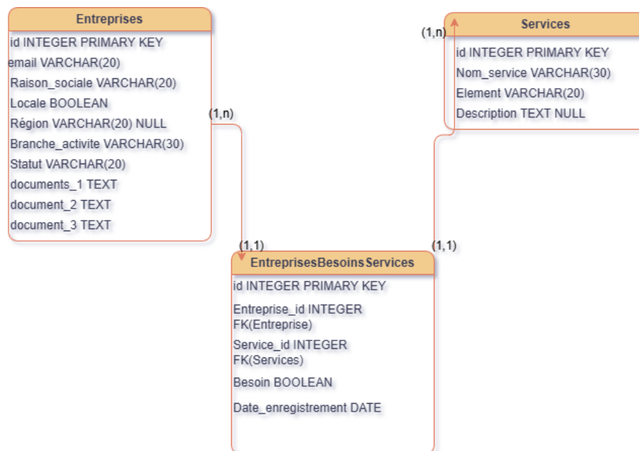
FIGURE 4.1 – Schéma de la base de données
