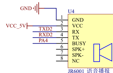
语音播报模块接口
