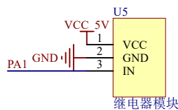
点火控制继电器
