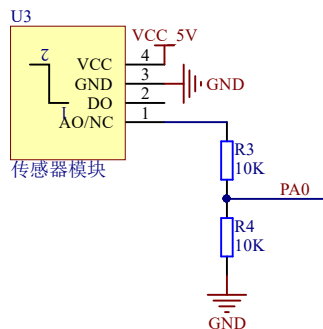
传感器模块
