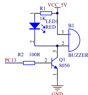
蜂鸣器报警
