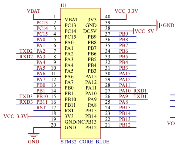
核心板
