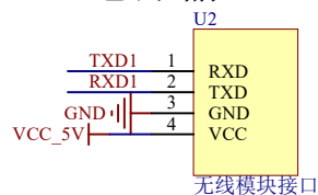
无线模块接口
