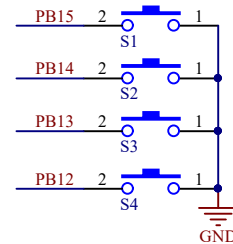
按键电路
