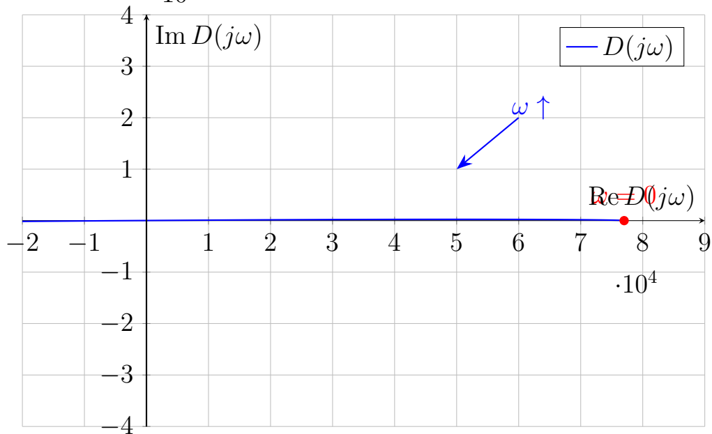
Рис. 3: Годограф Михайлова для устойчивой системы
