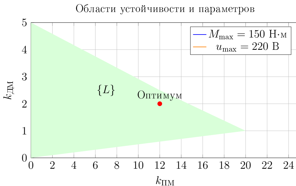
Рис. 4: Область устойчивости и допустимых параметров на плоскости (k_{\text{ПМ}}, k_{\text{ДМ}})
