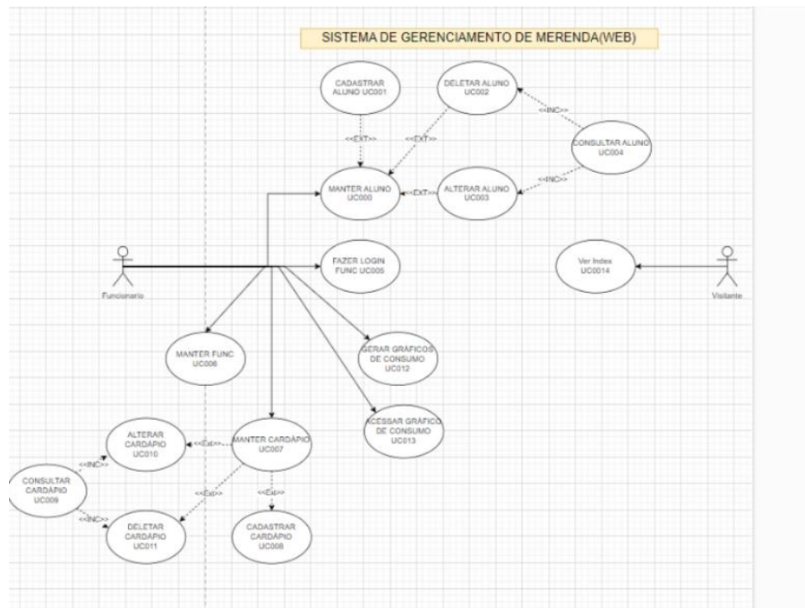
Figura 1 – Diagrama de caso de uso WEB
