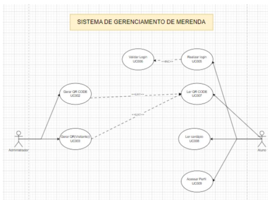
Figura 2 – Diagrama de caso de uso APP
