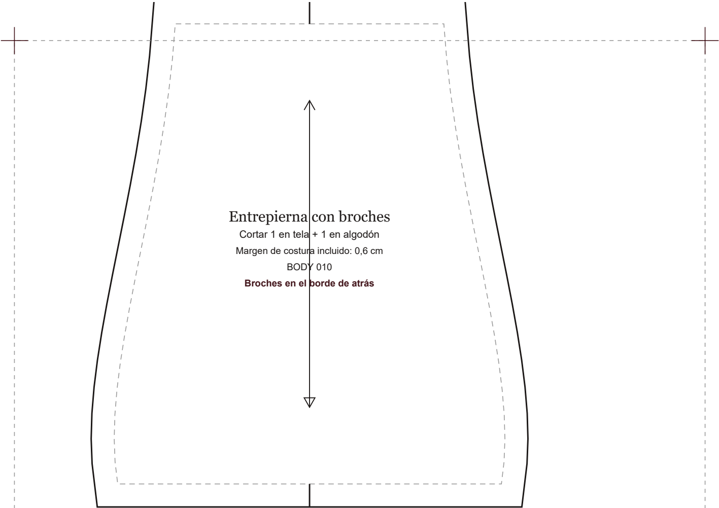
BODY 010 · Body Escote Cuadrado · Espalda Cavada · escala 1:1 · 104,6 × 88,3 cm
