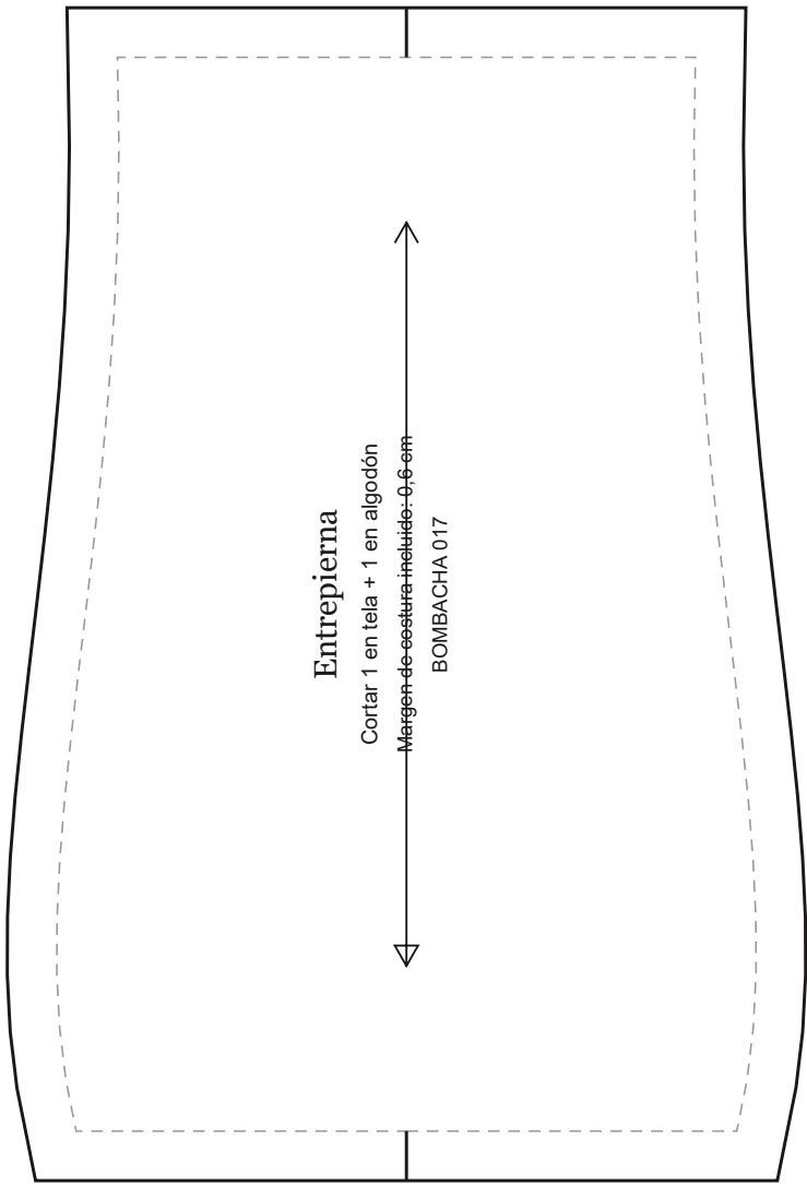
BOMBACHA 017 · Culotte de Tiro Alto · escala 1:1 · 62,8 × 68,1 cm
