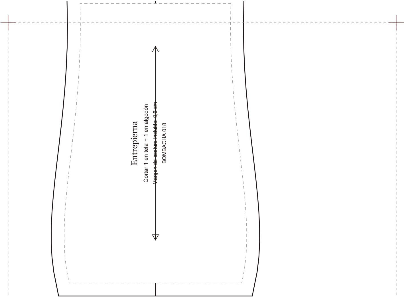
BOMBACHA 018 · Culotte con Pierna Recta · escala 1:1 · 62,8 × 64,1 cm
