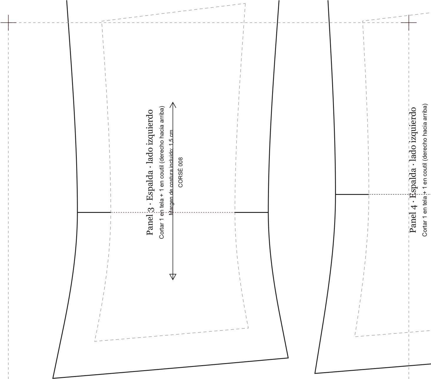
CORSÉ 008 · Cinturón Corsé · 5 Paneles · Borde Asimétrico · escala 1:1 · 94,6 × 42,7 cm
