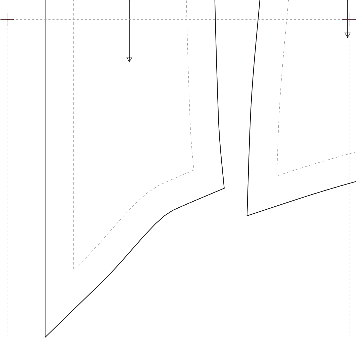
CORSÉ 048 · Bajo Busto Eduardiano de Frente Recto · 6 Paneles · Borde en Punta · escala 1:1 · 83,9 × 43,4 cm
