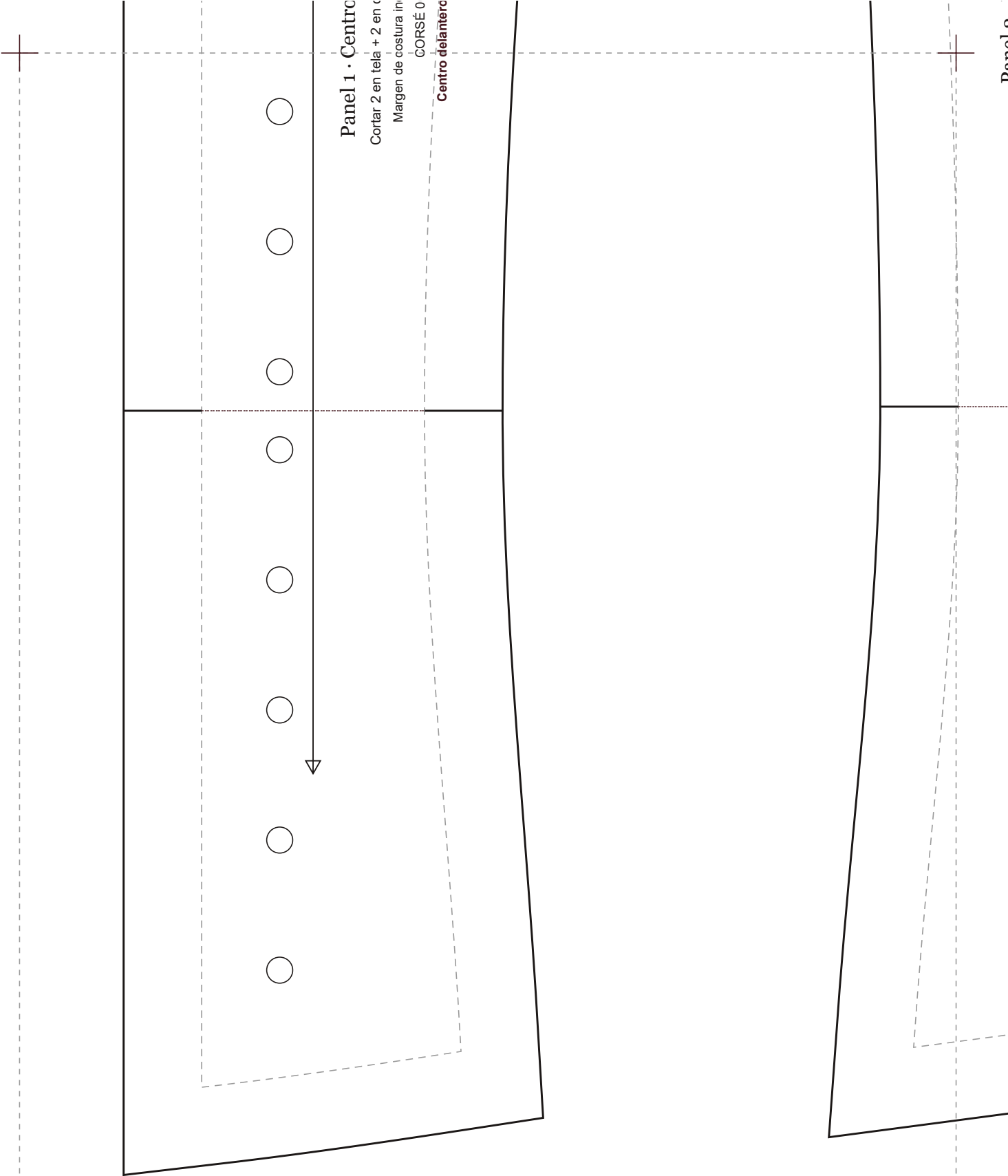
CORSÉ 066 · Sobre Busto Escote Recto · 7 Paneles · Cordón Adelante · escala 1:1 · 91 × 48,3 cm
