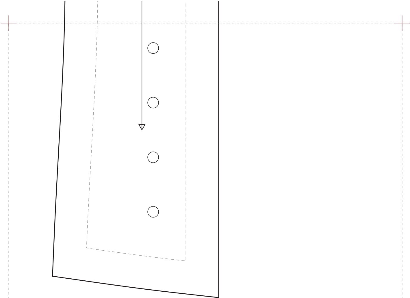
CORSÉ 067 · Sobre Busto Escote Recto · 8 Paneles · Busk · escala 1:1 · 88,7 × 88,7 cm
