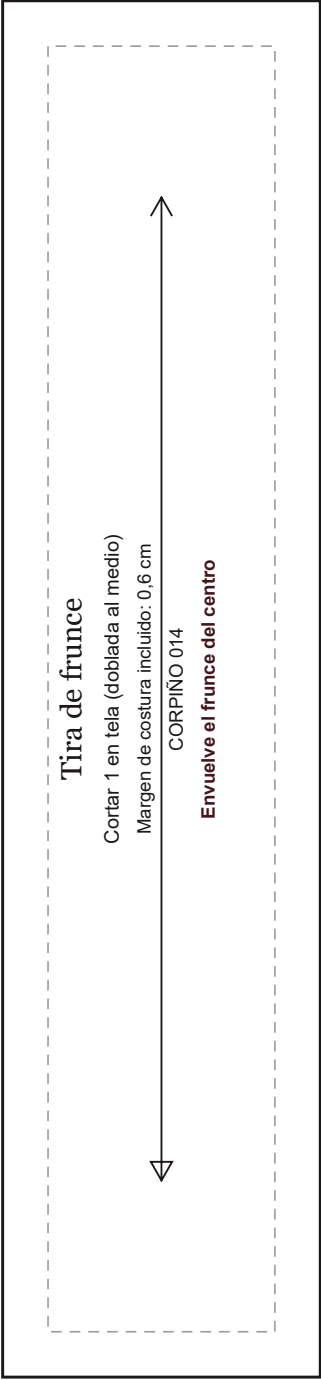
CORPIÑO 014 · Bandeau con Frunce Central · escala 1:1 · 93,9 × 45,9 cm
