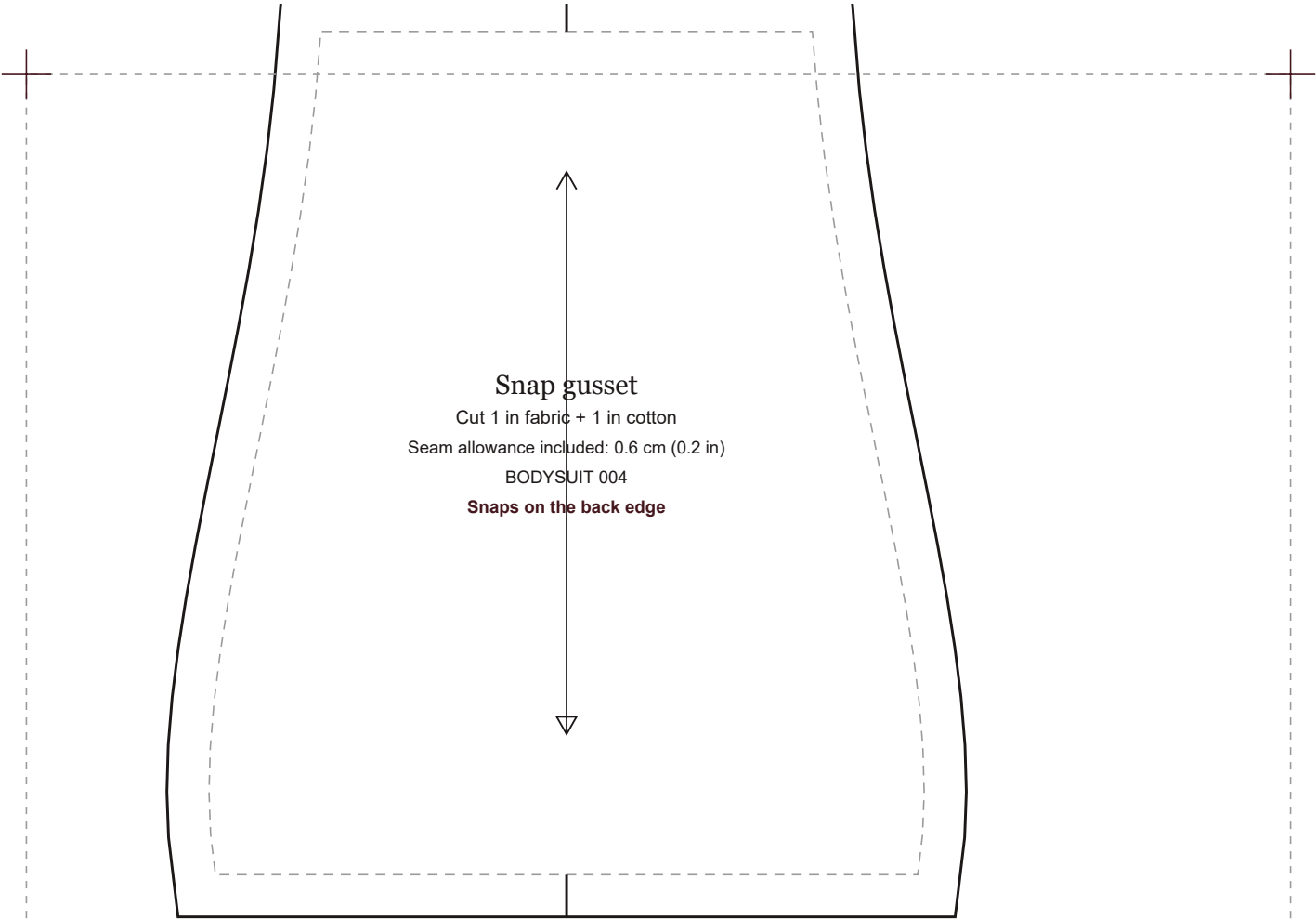
BODYSUIT 004 · Bodysuit · Round Neck · Keyhole Back · scale 1:1 · 104.6 × 88.1 cm (41.2 × 34.7 in)
