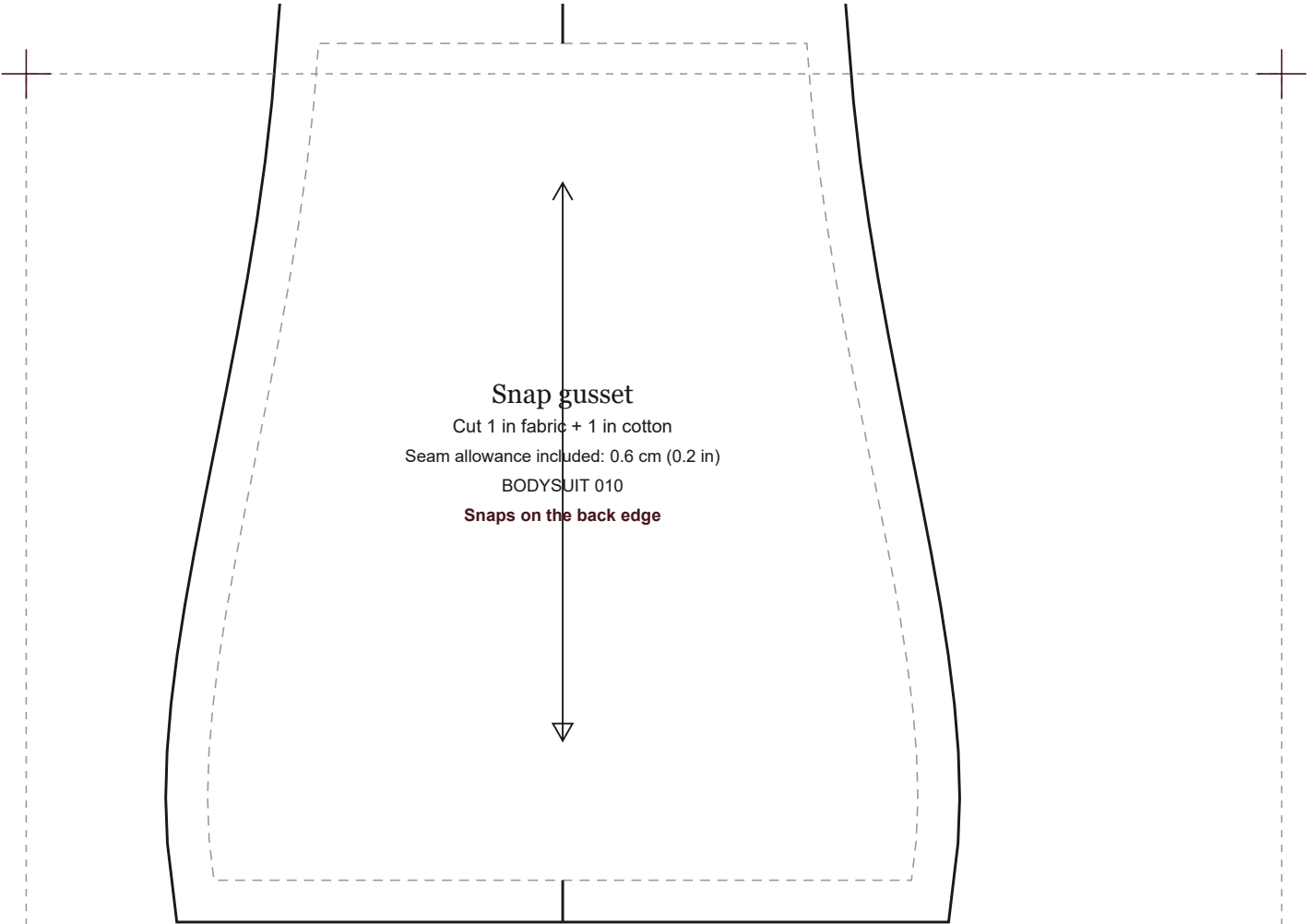
BODYSUIT 010 · Bodysuit · Square Neck · Low Back · scale 1:1 · 104.6 × 88.3 cm (41.2 × 34.7 in)
