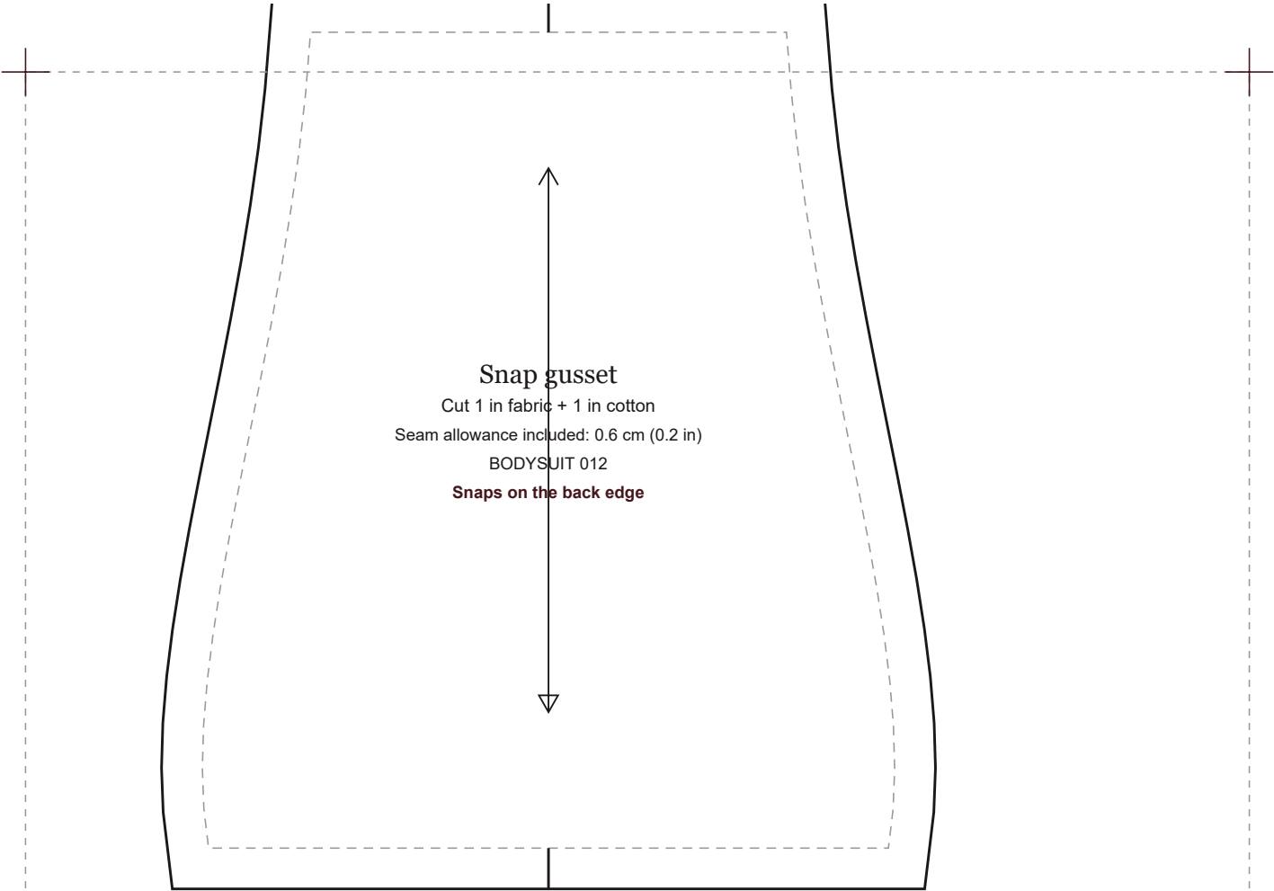
BODYSUIT 012 · Bodysuit · Square Neck · Keyhole Back · scale 1:1 · 104.6 × 88.1 cm (41.2 × 34.7 in)
