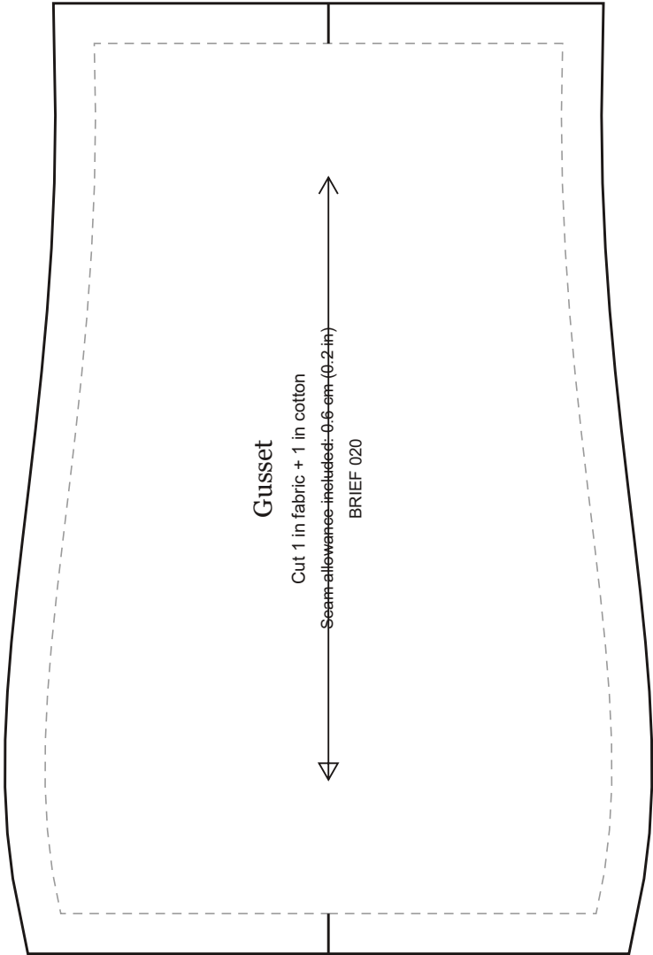
BRIEF 020 · Long-Leg Boyshort · scale 1:1 · 62.8 × 66.3 cm (24.7 × 26.1 in)
