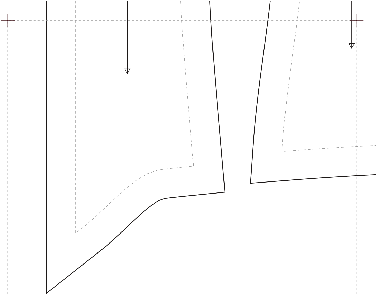
CORSET 026 · Classic Underbust · 6 Panels · Pointed Edge · scale 1:1 · 83.3 × 40.8 cm (32.8 × 16.1 in)
