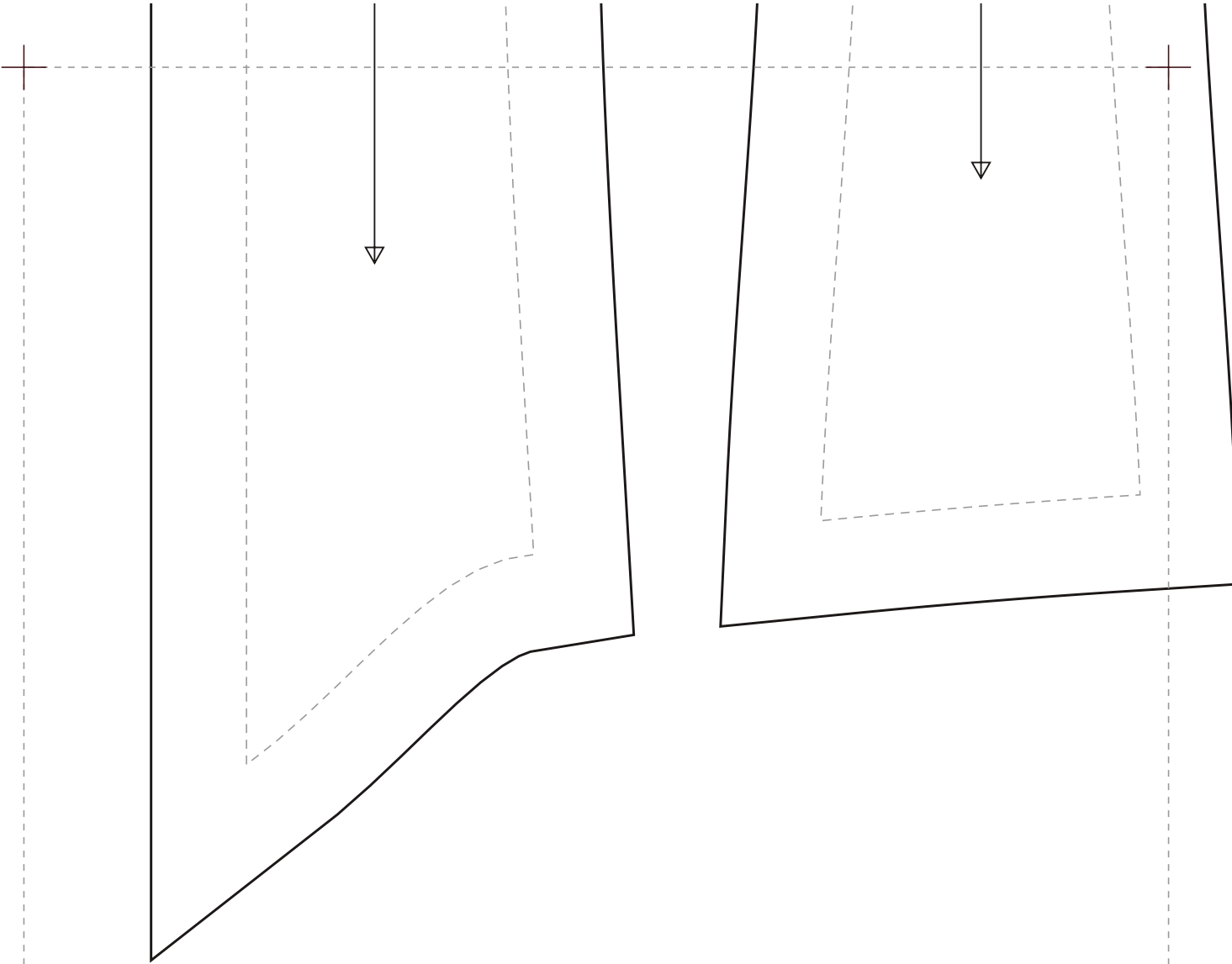
CORSET 034 · Classic Underbust · 8 Panels · Pointed Edge · scale 1:1 · 91.8 × 40.8 cm (36.1 × 16.0 in)
