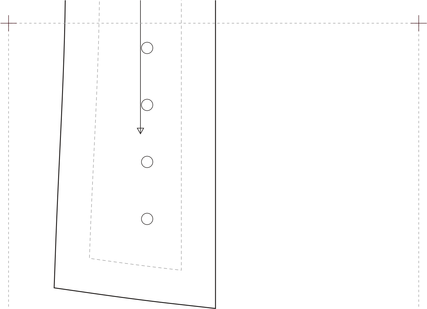
CORSET 069 · Straight-Neckline Overbust · 9 Panels · Busk · scale 1:1 · 93.4 × 88.6 cm (36.8 × 34.9 in)
