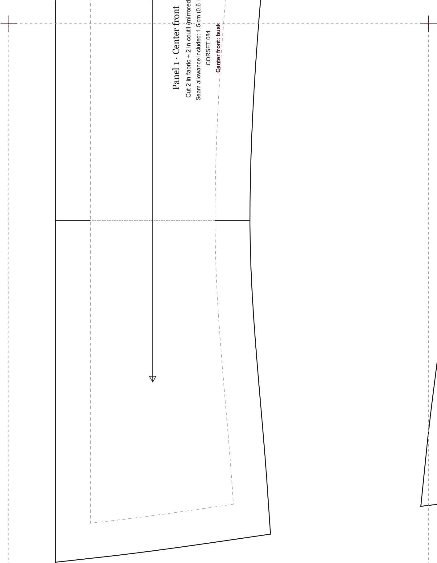
CORSET 084 · Deep V-Neck Overbust · 6 Panels · scale 1:1 · 89.5 × 49.8 cm (35.2 × 19.6 in)
