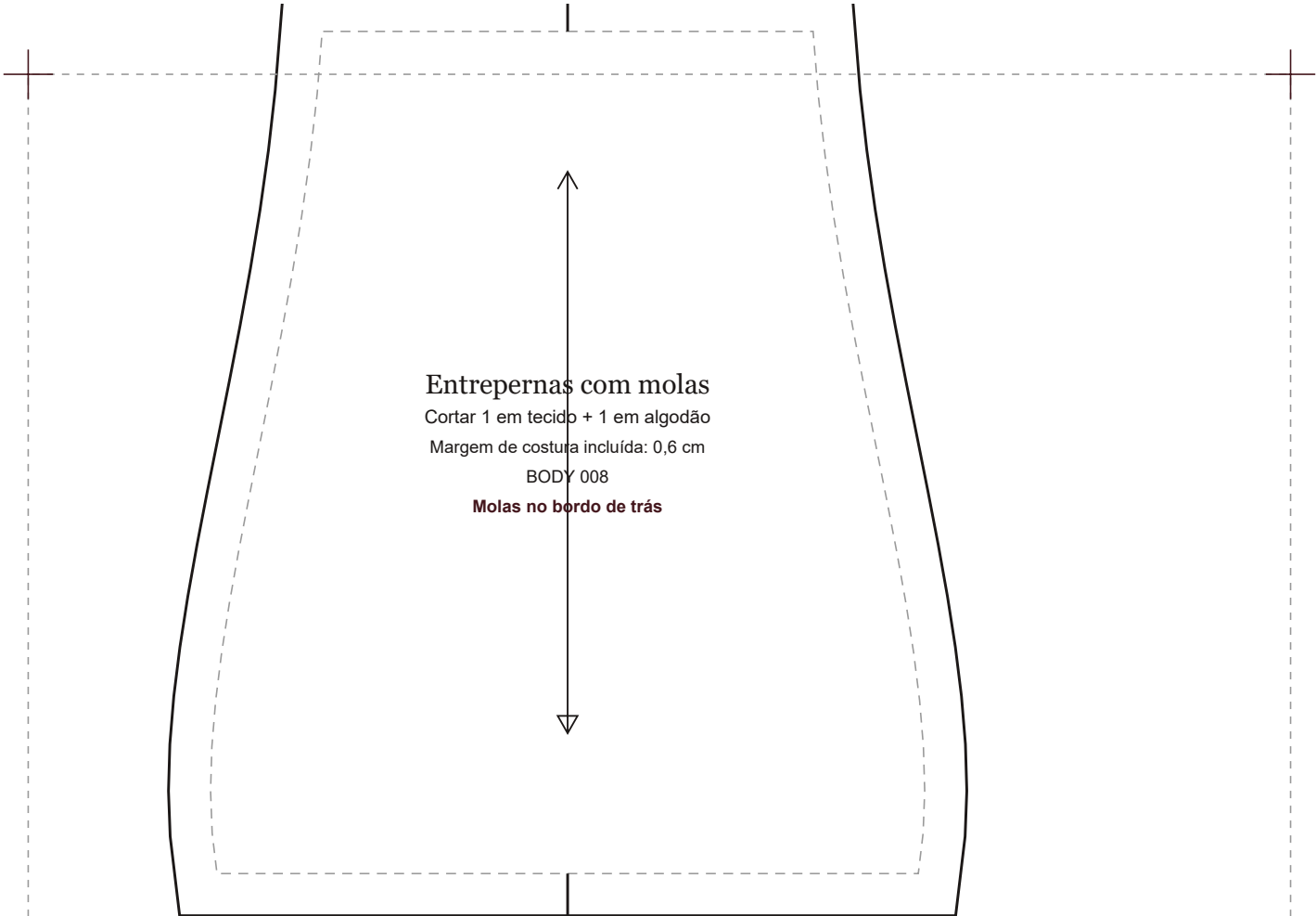
BODY 008 · Body com Decote em V · Costas Abertas em Gota · escala 1:1 · 104,6 × 88,1 cm
