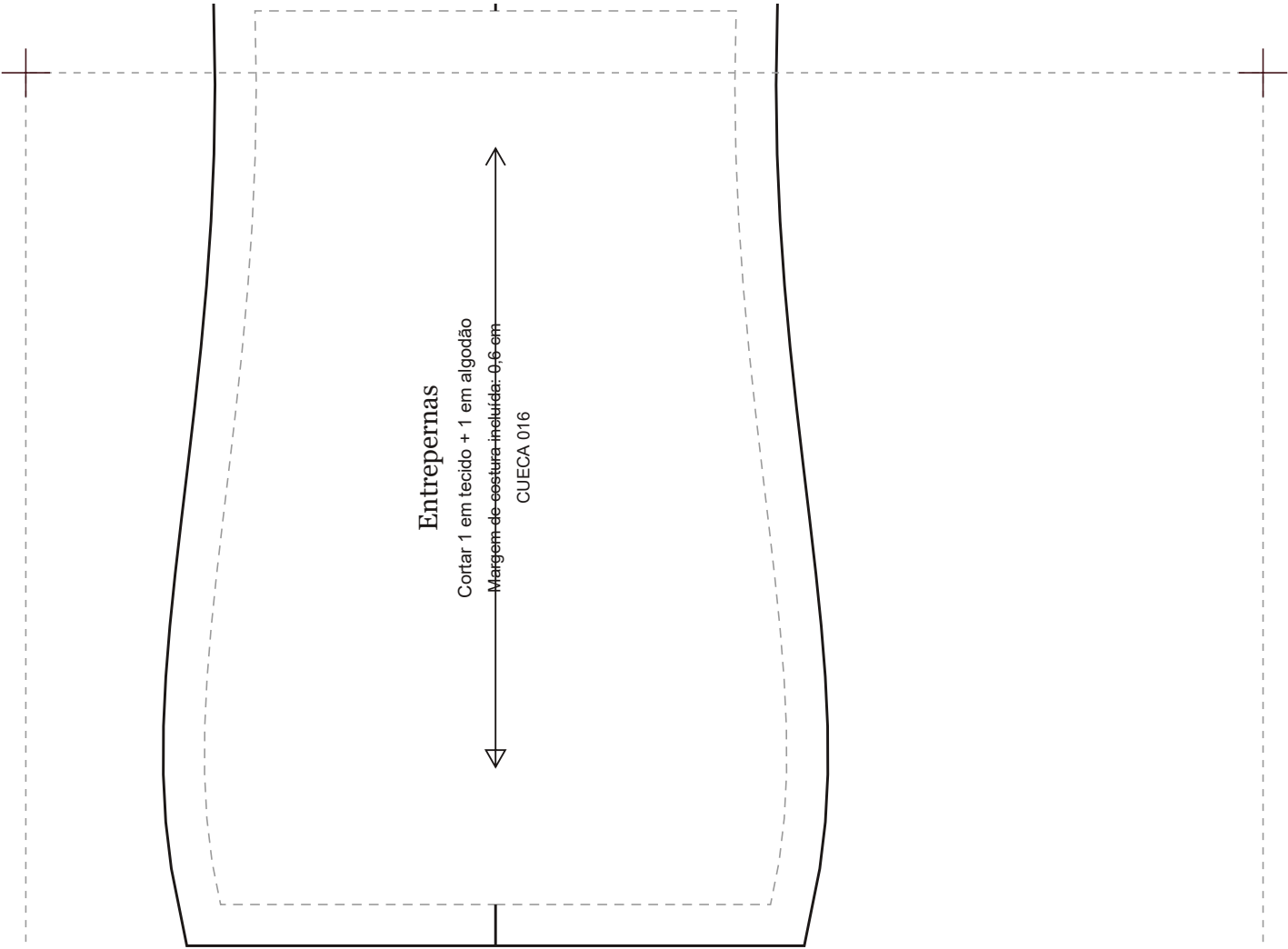
CUECA 016 · Culotte Clássico · escala 1:1 · 62,8 × 64,1 cm
