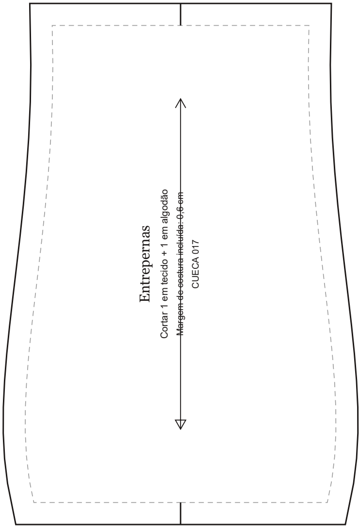
CUECA 017 · Culotte de Cintura Subida · escala 1:1 · 62,8 × 68,1 cm
