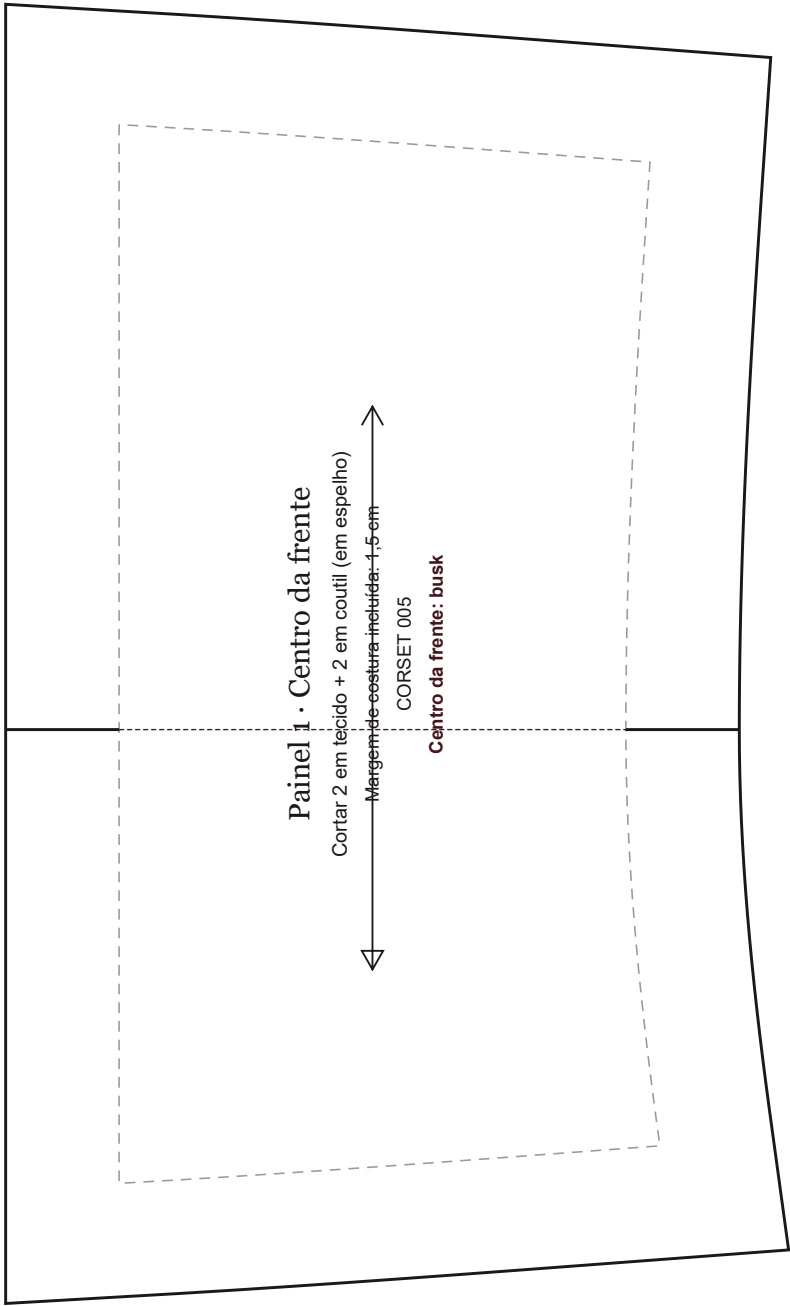
CORSET 005 · Cinto Corset · 5 Painéis · Bordo Reto · escala 1:1 · 71,3 × 21,2 cm
