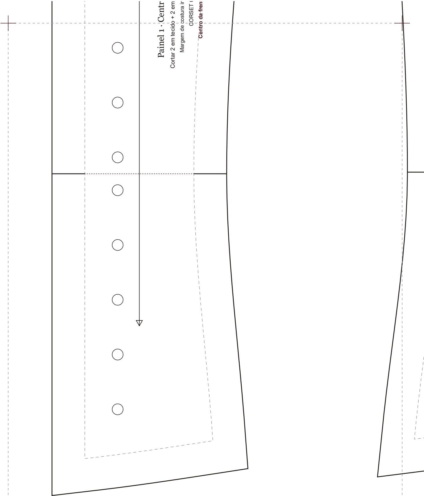
CORSET 064 · Sobre o Busto com Decote Reto · 6 Painéis · Atacador à Frente · escala 1:1 · 86,9 × 48,3 cm
