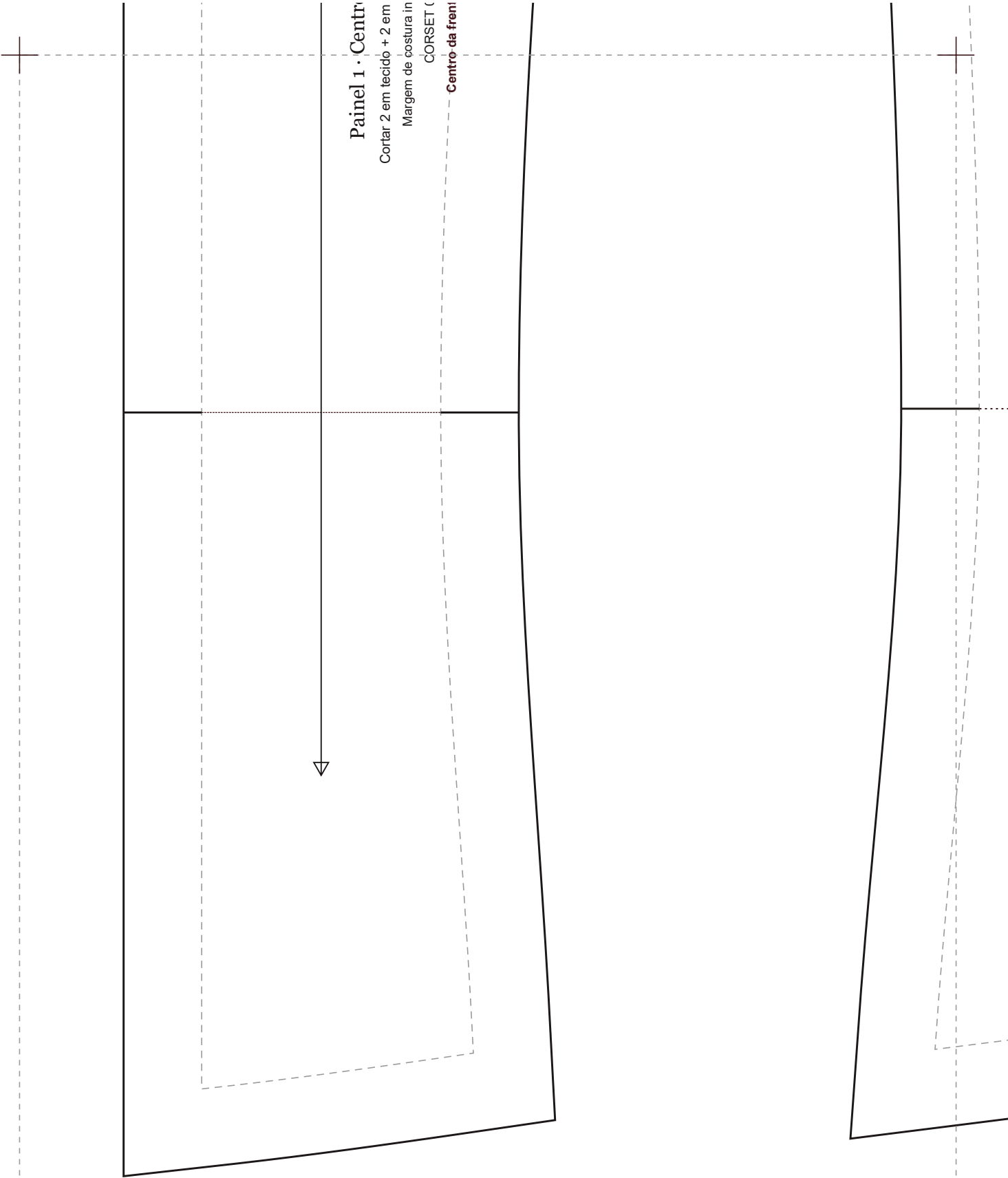
CORSET 065 · Sobre o Busto com Decote Reto · 7 Painéis · Busk · escala 1:1 · 93,2 × 48,2 cm
