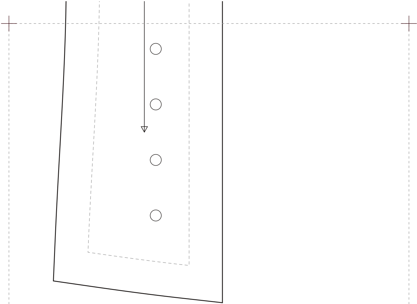
CORSET 067 · Sobre o Busto com Decote Reto · 8 Painéis · Busk · escala 1:1 · 88,7 × 88,7 cm
