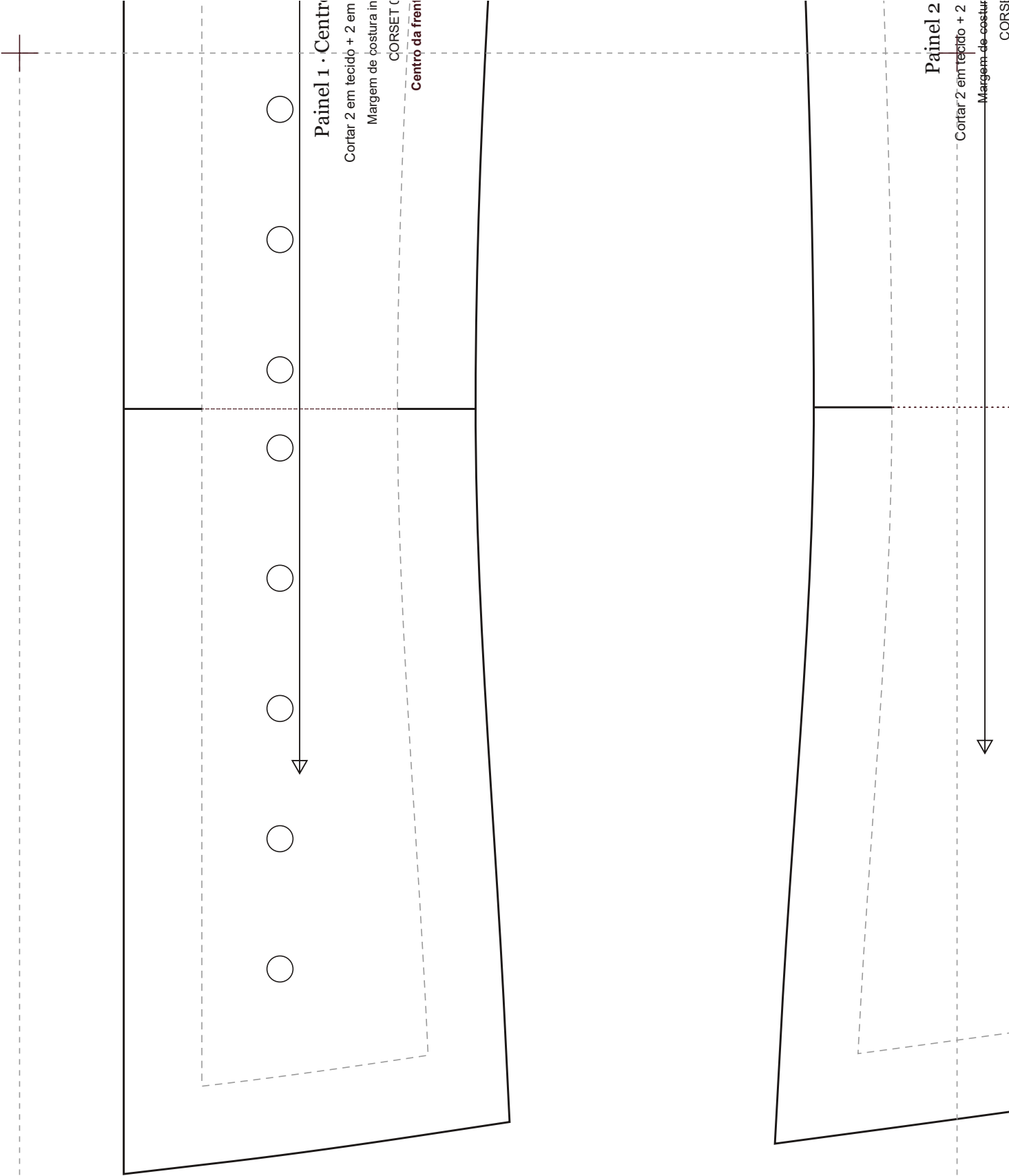
CORSET 068 · Sobre o Busto com Decote Reto · 8 Painéis · Atacador à Frente · escala 1:1 · 95,3 × 48,2 cm
