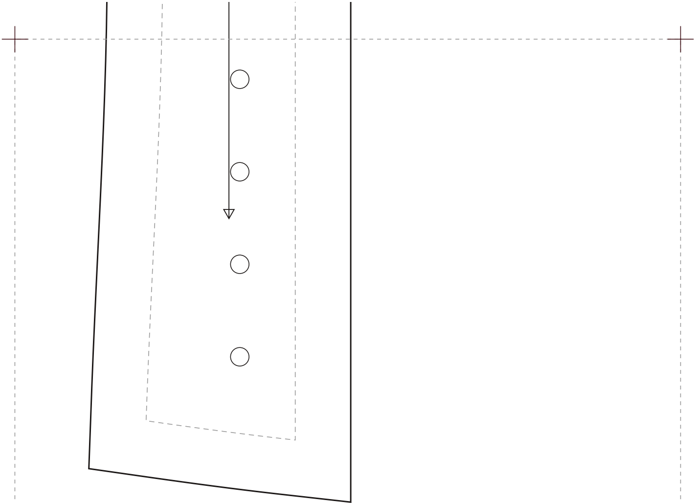
CORSET 069 · Sobre o Busto com Decote Reto · 9 Painéis · Busk · escala 1:1 · 93,4 × 88,6 cm
