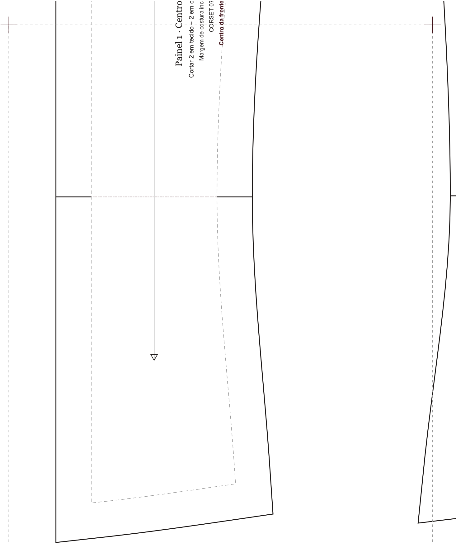
CORSET 073 · Sobre o Busto com Decote Coração · 6 Painéis · Bordo Reto · escala 1:1 · 89,2 × 48,7 cm
