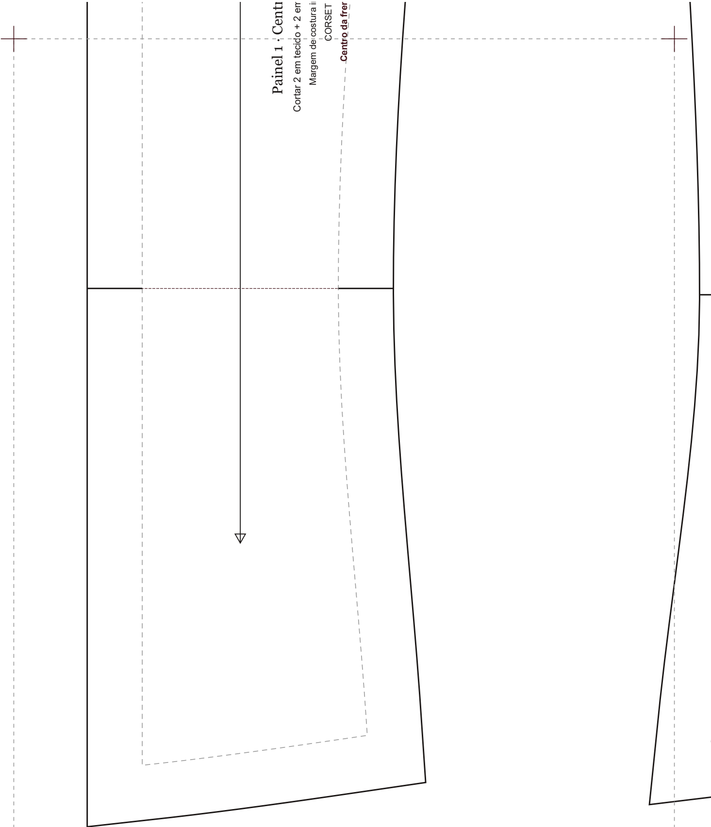
CORSET 083 · Sobre o Busto com Decote em V Suave · 6 Painéis · escala 1:1 · 89,1 × 48,2 cm
