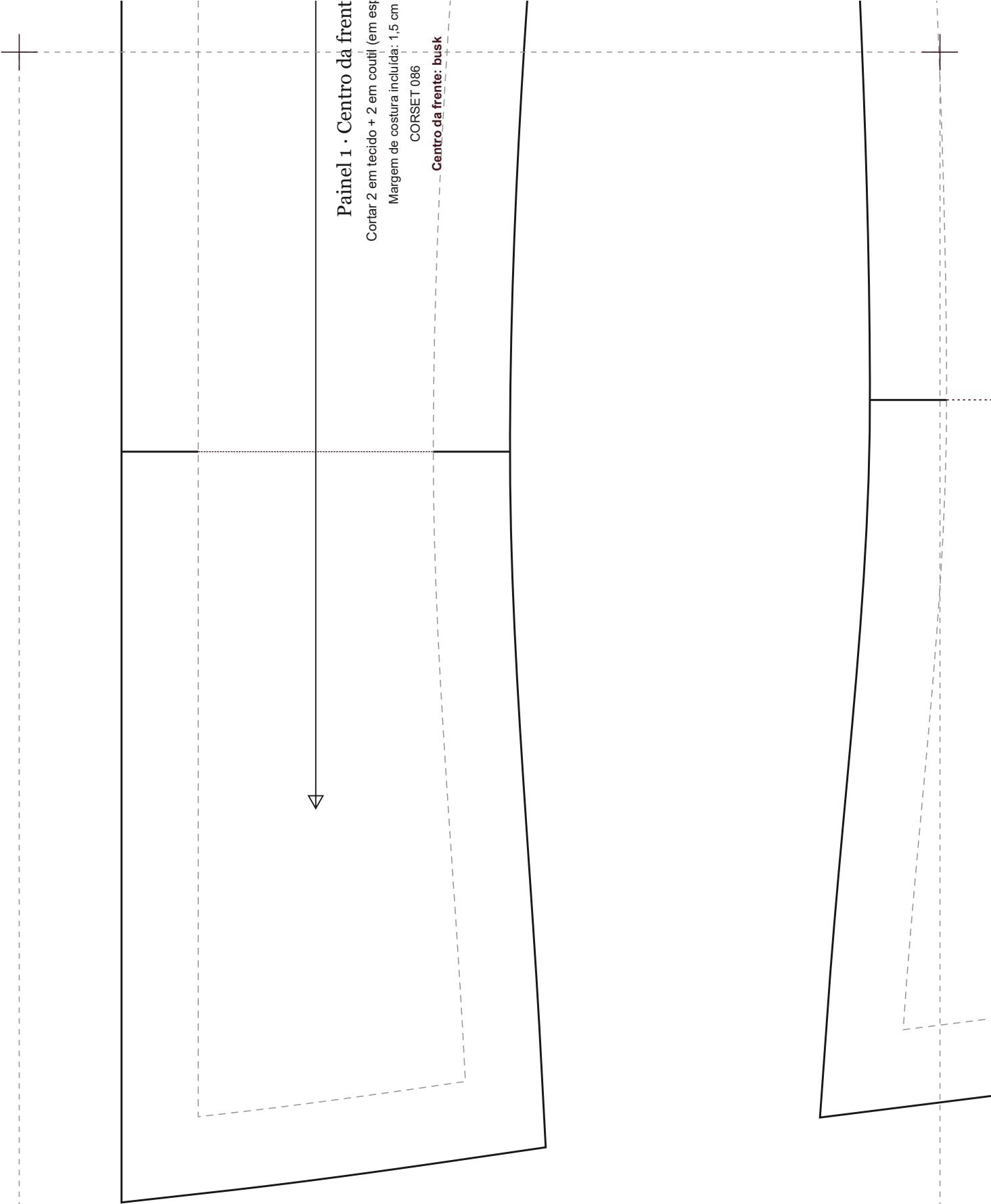
CORSET 086 · Sobre o Busto com Decote em V Profundo · 7 Painéis · escala 1:1 · 92,9 × 49,2 cm
