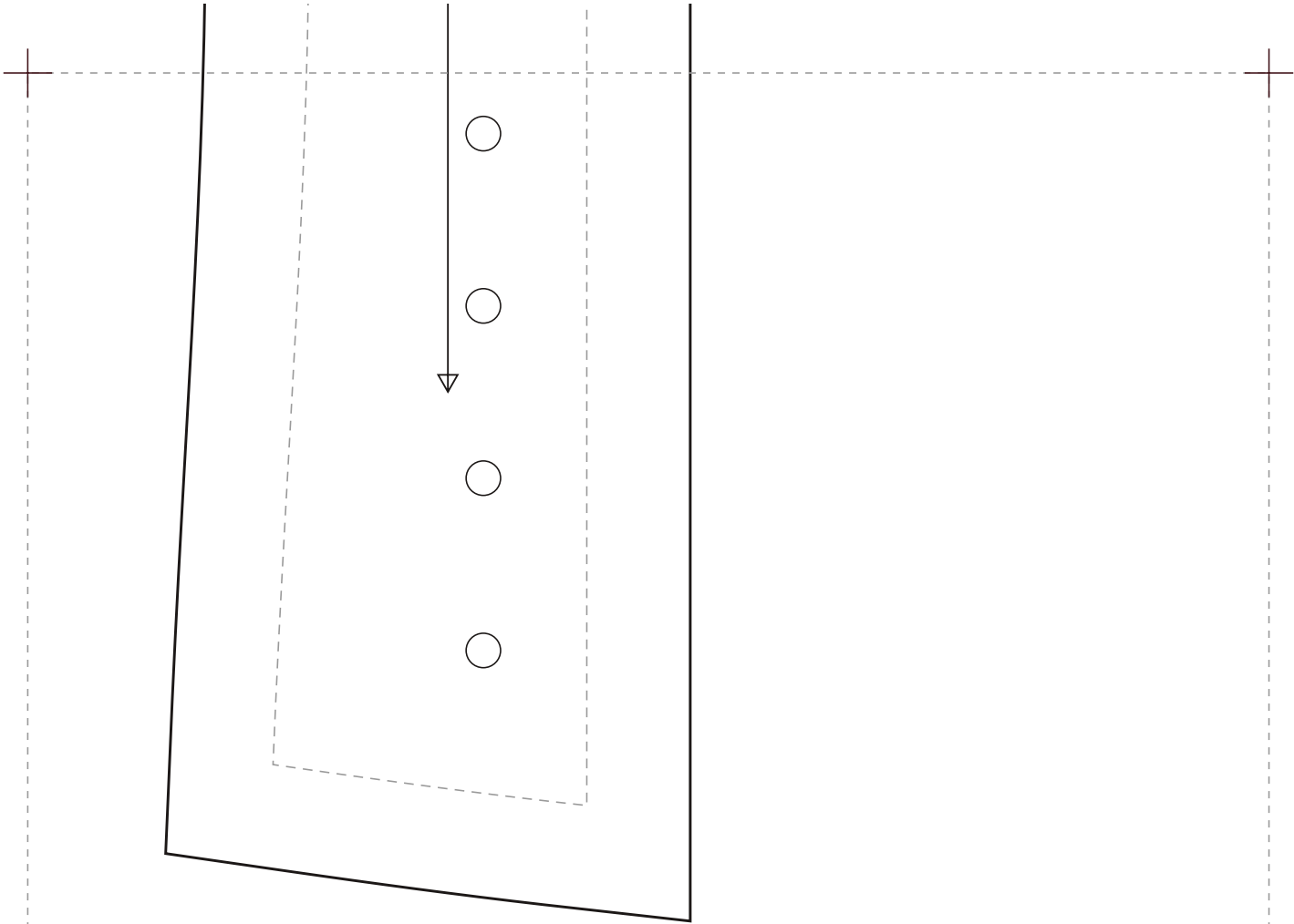
CORSET 088 · Sobre o Busto com Decote em V Profundo · 8 Painéis · escala 1:1 · 87,9 × 88,4 cm
