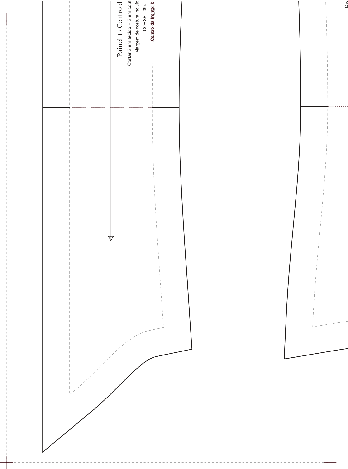
CORSET 094 · Sobre o Busto Balconete · 7 Painéis · Bordo em Bico · escala 1:1 · 92 × 50,8 cm
