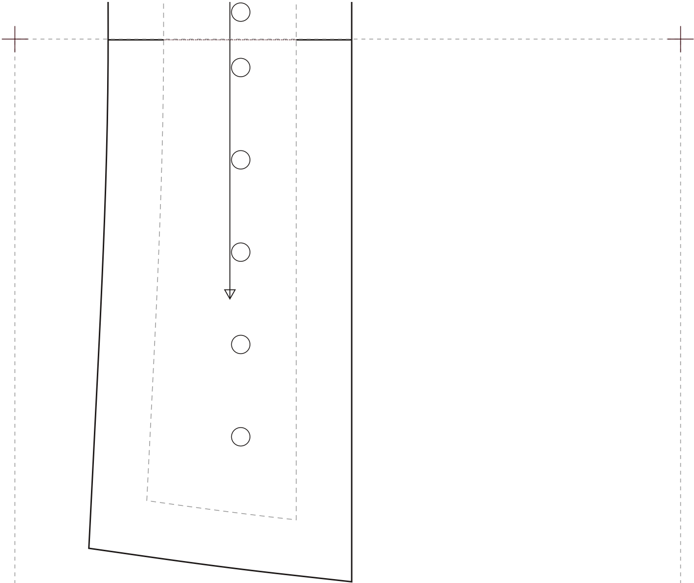
CORSET 098 · Sobre o Busto Balconete · 9 Painéis · Bordo em Bico · escala 1:1 · 92,2 × 90,8 cm
