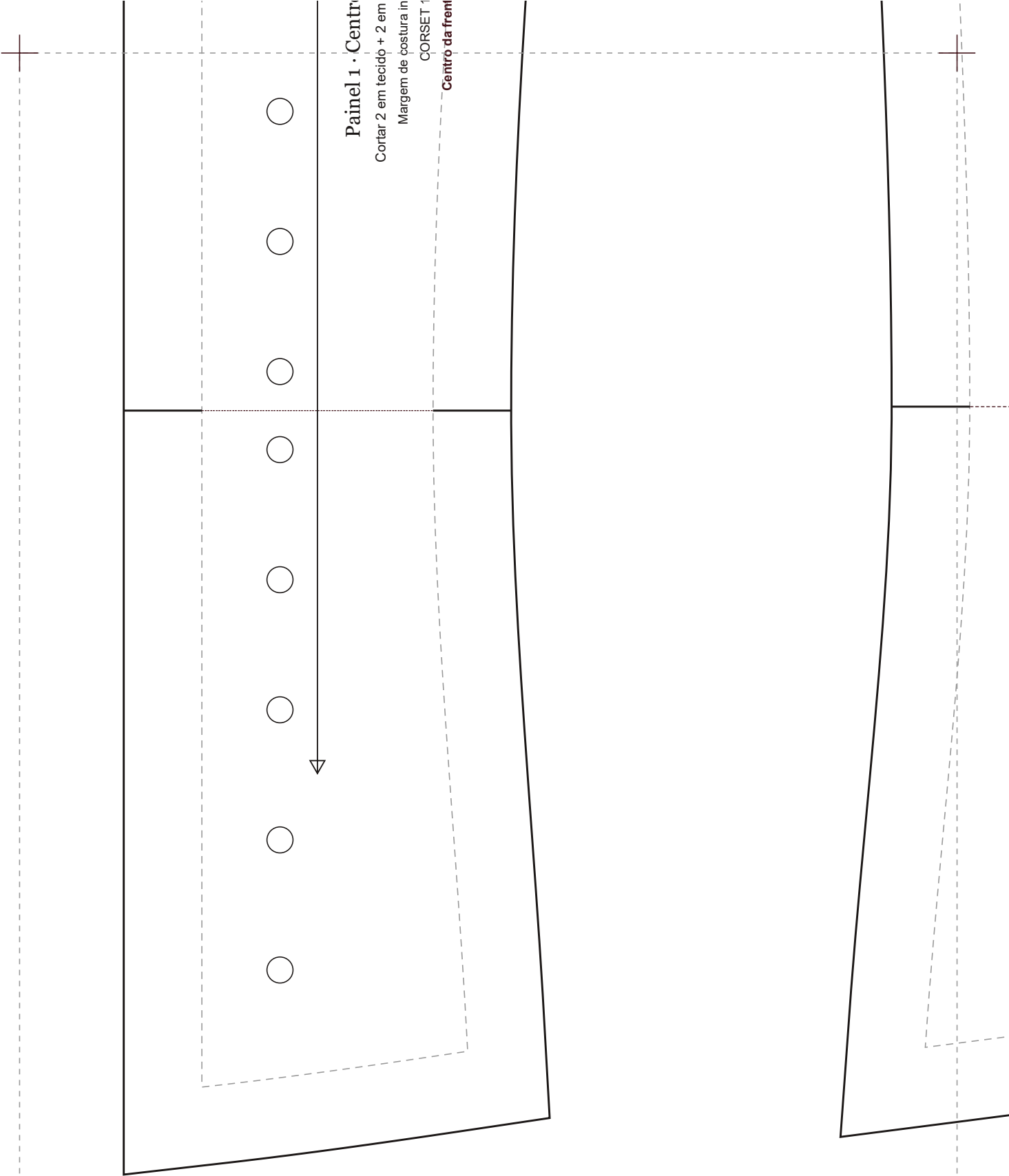
CORSET 108 · Sobre o Busto com Atacador à Frente e Atrás · 7 Painéis · escala 1:1 · 92,1 × 48,3 cm
