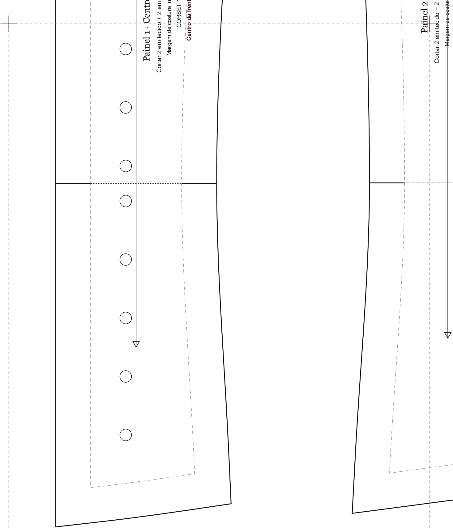
CORSET 110 · Sobre o Busto com Atacador à Frente e Atrás · 8 Painéis · escala 1:1 · 96,4 × 48,2 cm
