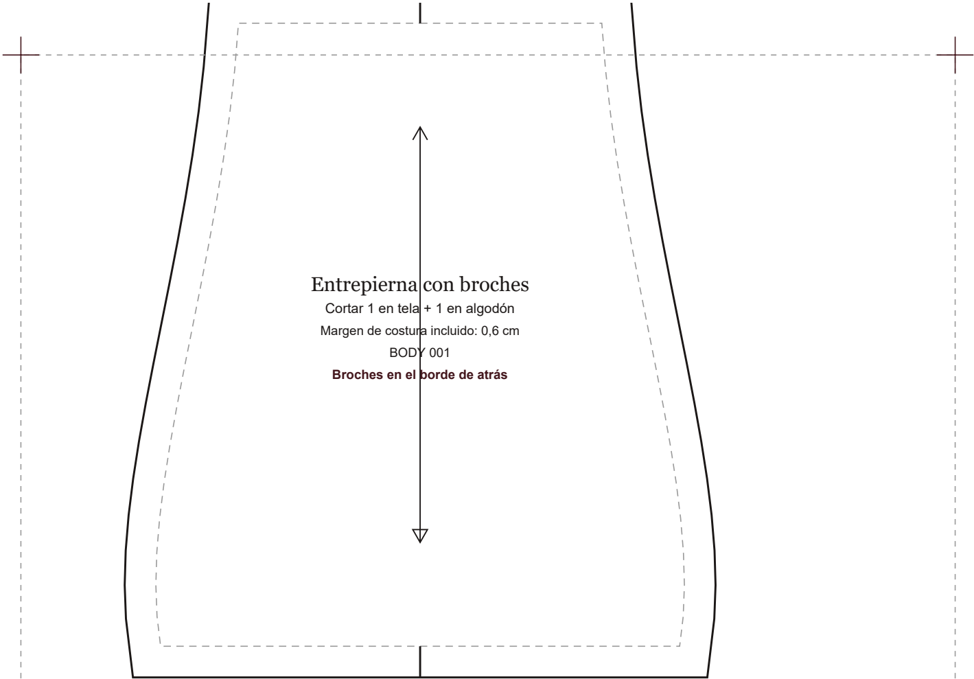
BODY 001 · Body Escote Redondo · Espalda Cerrada · escala 1:1 · 104,6 × 88,1 cm
