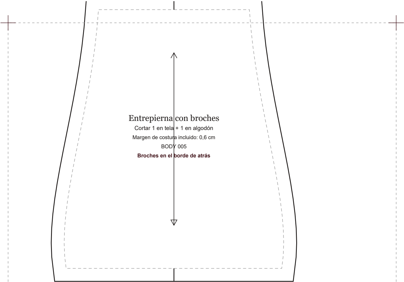
BODY 005 · Body Escote en V · Espalda Cerrada · escala 1:1 · 104,6 × 88,1 cm
