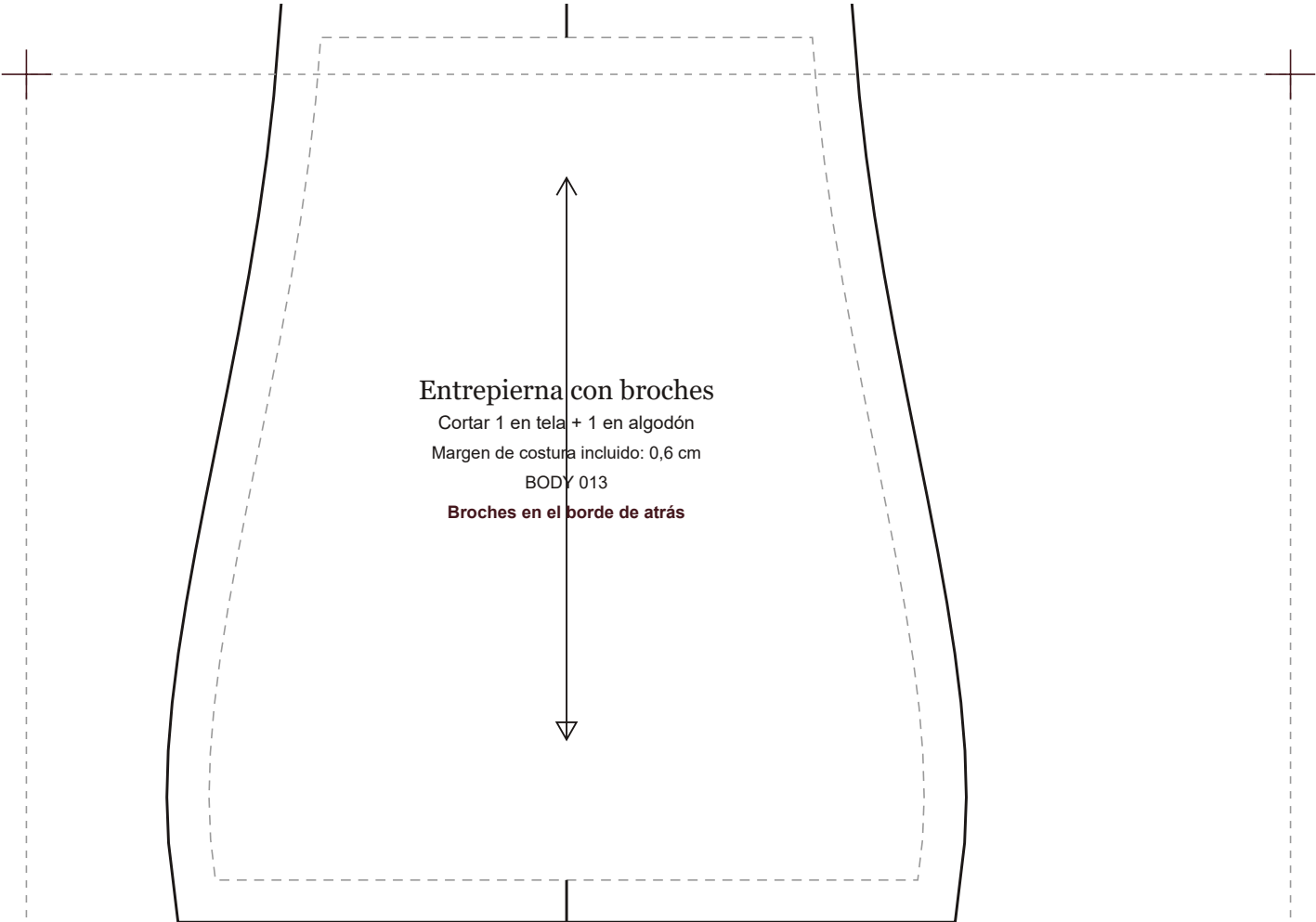
BODY 013 · Body Escote Corazón · Espalda Cerrada · escala 1:1 · 104,6 × 88,2 cm
