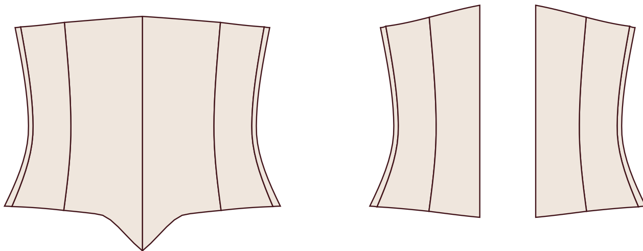
DIBUJO TÉCNICO (sale del mismo trazado)
