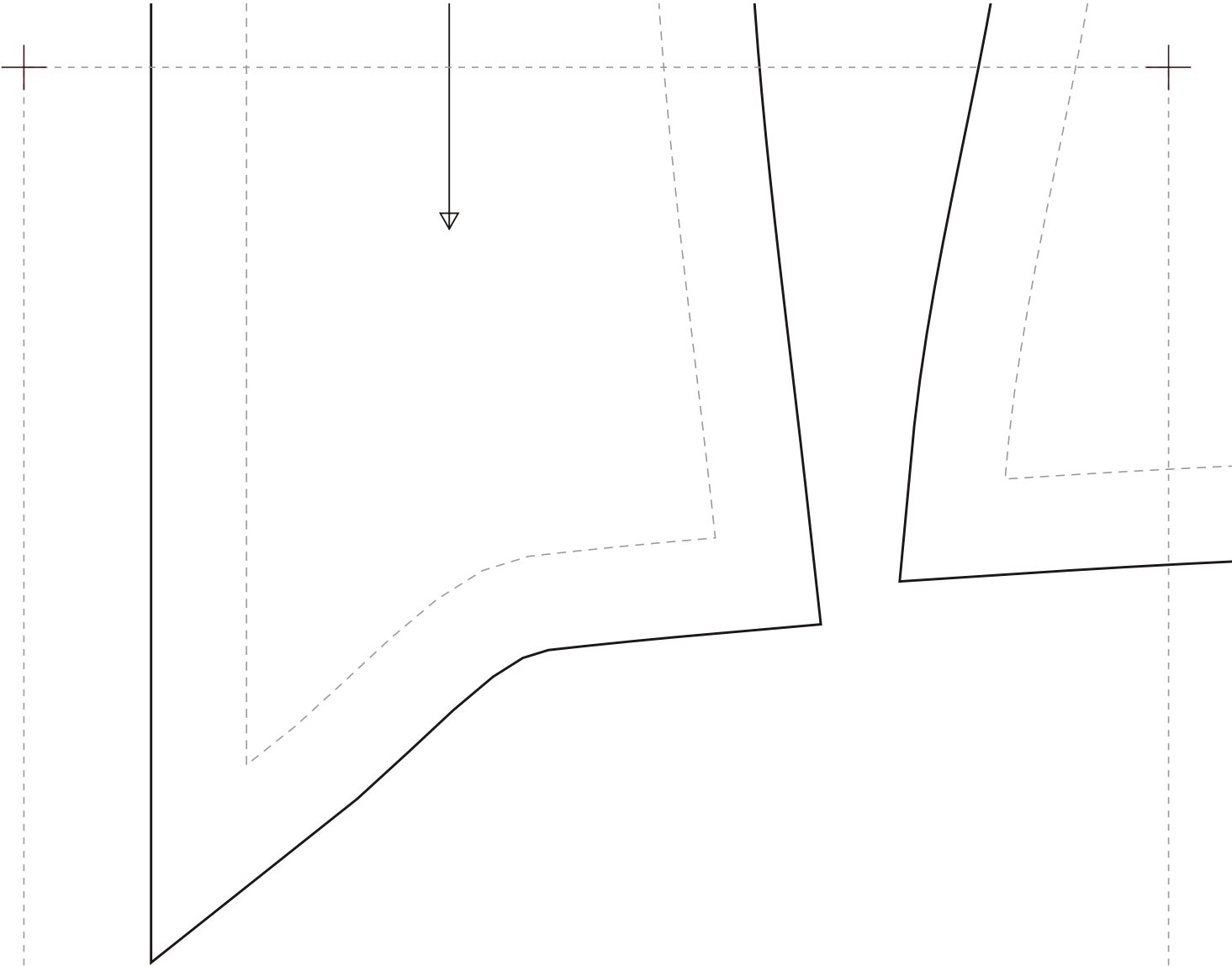
CORSÉ 022 · Bajo Busto Clásico · 5 Paneles · Borde en Punta · escala 1:1 · 78,9 × 40,8 cm
